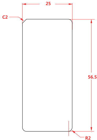
尺寸图
