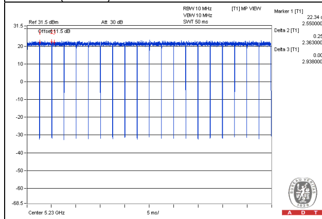
802.11n (40MHz)
