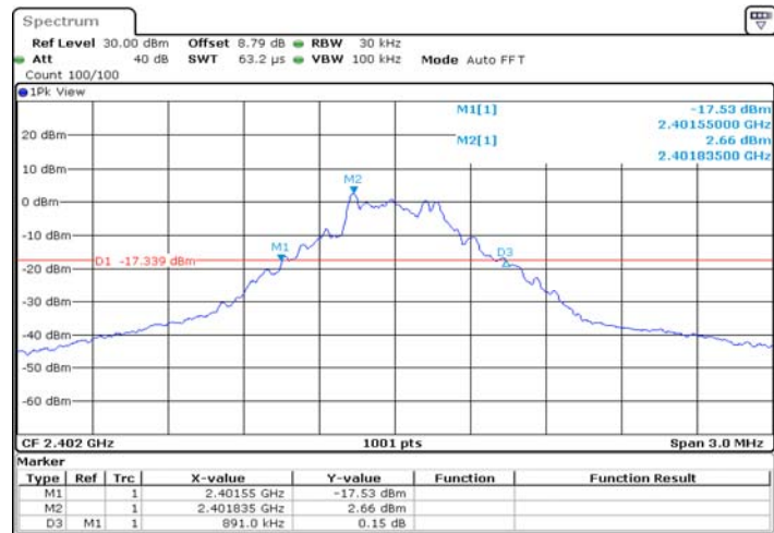
DH1_Ant1_2402
