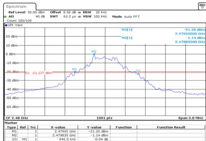
DH1_Ant1_2480
