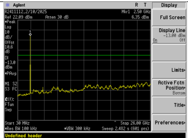
High Ch_2480MHz_2DH1_-20dBc_30MHz-26GHz
