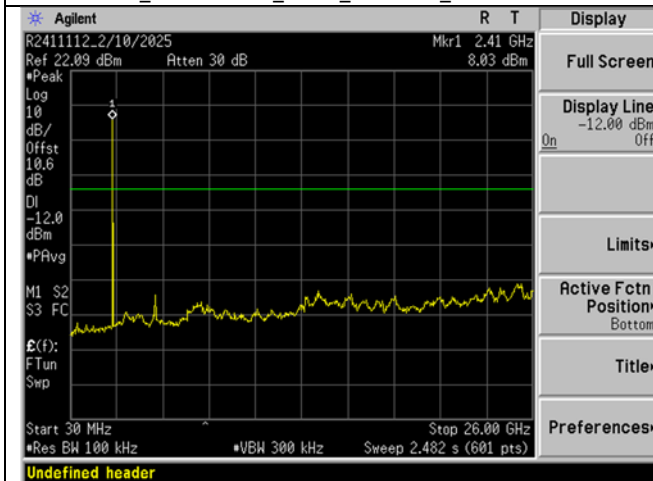
Low Ch_2402MHz_2DH1_-20dBc_30MHz-26GHz
