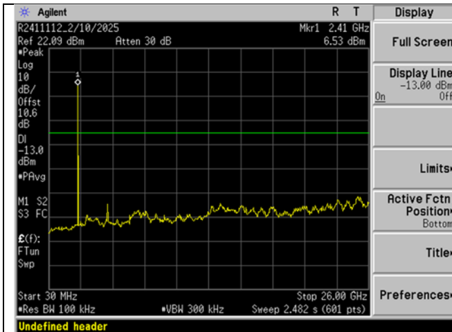
Low Ch_2402MHz_DH1_-20dBc_30MHz-26GHz
