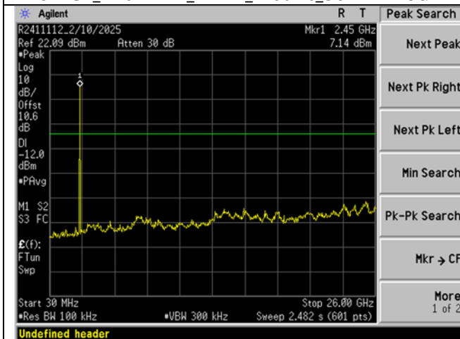
Mid Ch_2441MHz_2DH1_-20dBc_30MHz-26GHz
