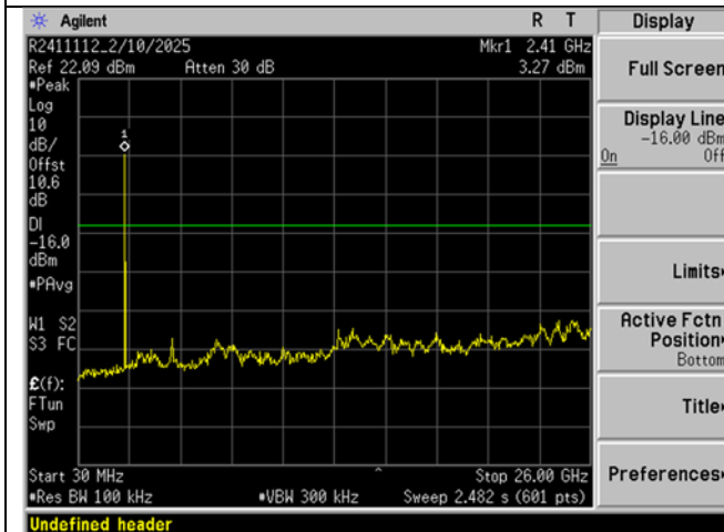
Low Ch_2402MHz_3DH1_-20dBc_30MHz-26GHz
