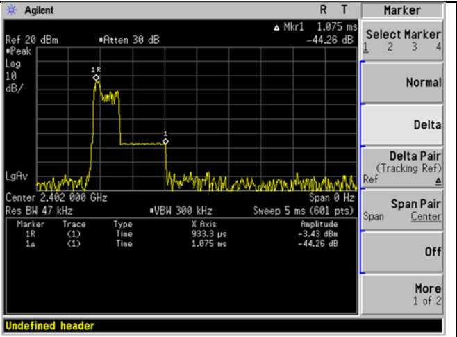
\pi/4 -DQPSK dwell time
