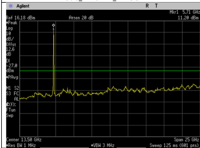
U-NII-2C_5720MHz_High Ch_144_20MHz BW_n/ac-mode_-27dBm_1-26GHz
