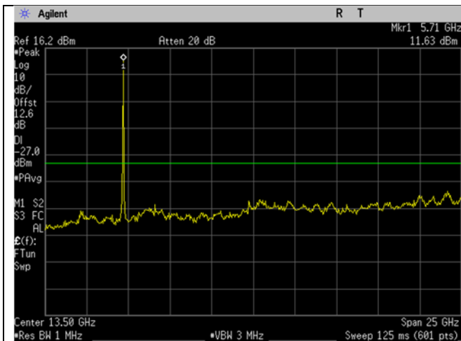
U-NII-2C_5700MHz_High Ch_140_20MHz BW_a-mode_-27dBm_1-26GHz
