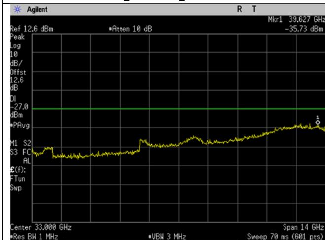
U-NII-1_5200MHz_low_Mid Ch_40_20MHz BW_n/ac-mode_-27dBm_26-40GHz
