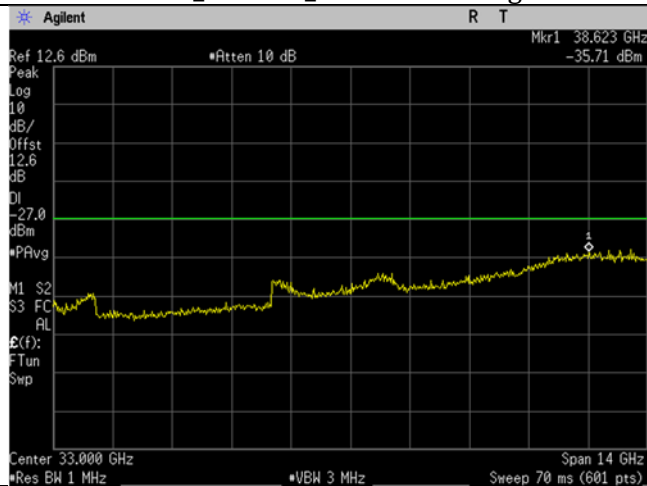
U-NII-2C_5530MHz_Low Ch_106_80MHz BW_ac-mode_-27dBm_26-40GHz
