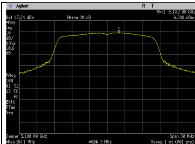
U-NII-1_5180MHz_Low Ch_36_20MHz BW_a-mode_Spectral Density
