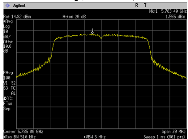
U-NII-3_5785MHz_Mid Ch_157_20MHz BW_a-mode_Spectral Density
