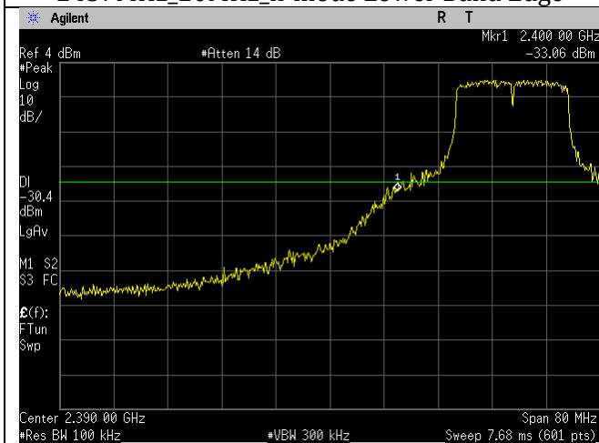
2417MHz_20MHz_g-mode_Lower Band Edge
