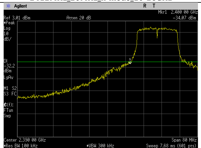
2412MHz_20MHz_n-mode_Lower Band Edge
