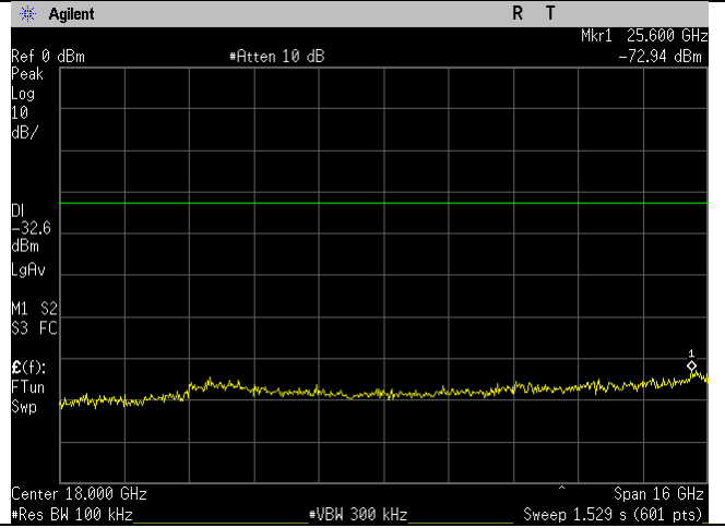
2462MHz_20MHz_g-mode_10-26GHz
