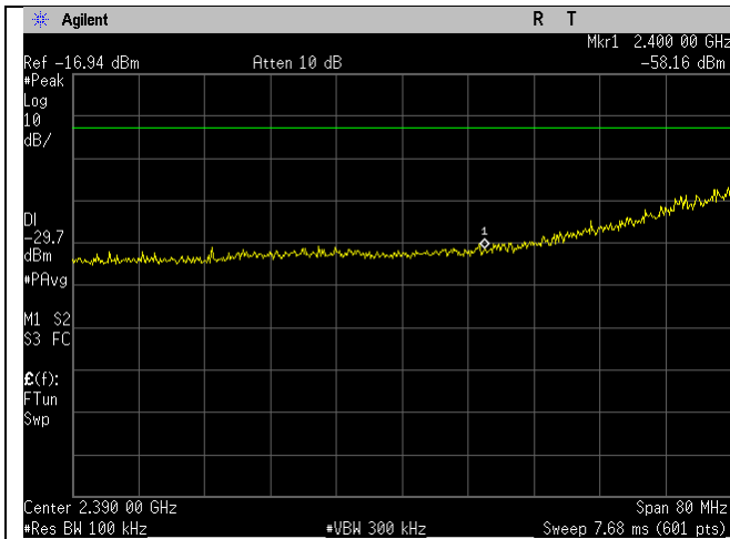
2457MHz_20MHz_g-mode_Lower Band Edge
