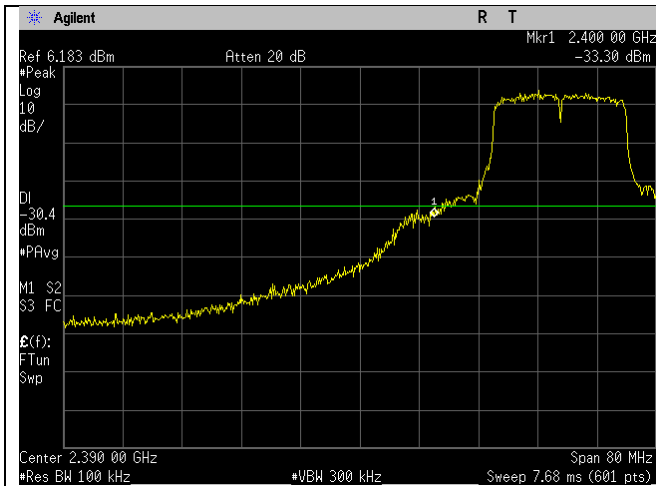
2417MHz_20MHz_n-mode_Lower Band Edge
