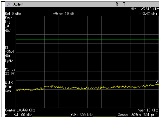
2437MHz_20MHz_g-mode_10-26GHz
