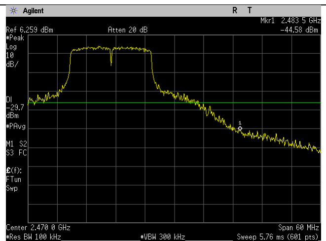
2457MHz_20MHz_g-mode_Upper Band Edge
