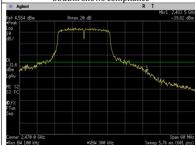
2462MHz_20MHz_n-mode_Upper Band Edge
