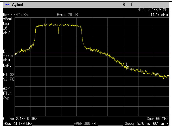
2457MHz_20MHz_n-mode_Upper Band Edge
