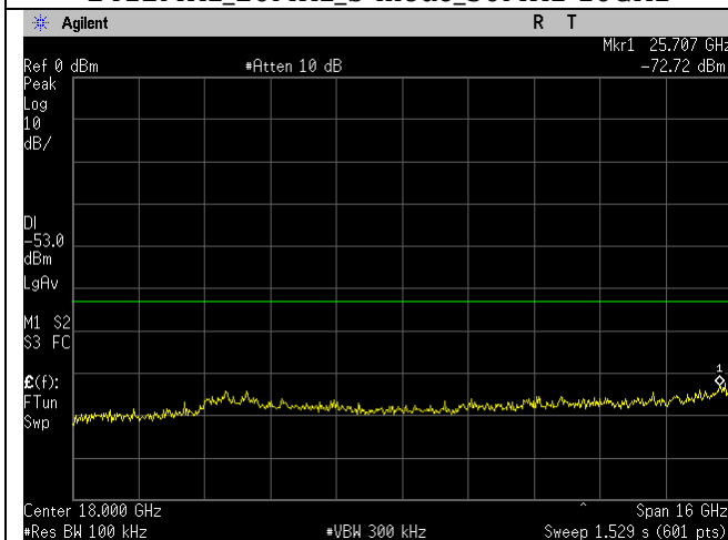
2412MHz_20MHz_g-mode_10-26GHz
