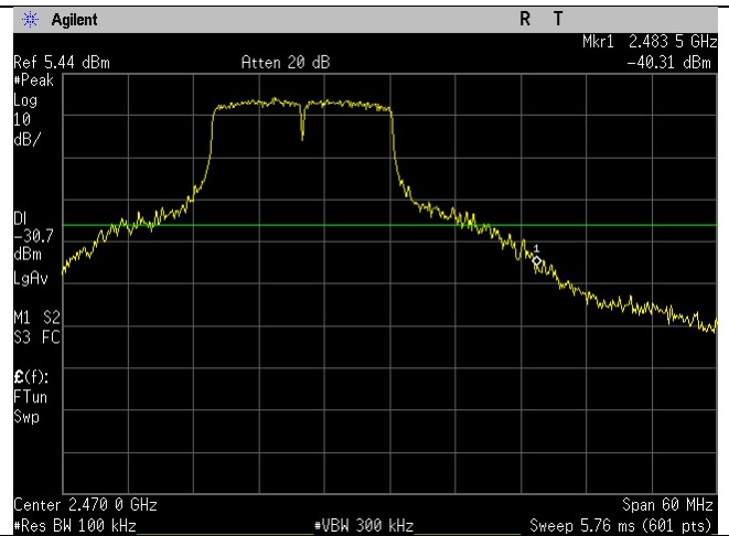
2462MHz_20MHz_g-mode_Upper Band Edge
