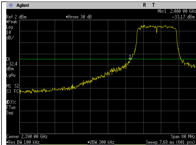
2412MHz_20MHz_g-mode_Lower Band Edge
