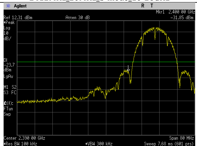
2412MHz_20MHz_b-mode_Lower Band Edge
