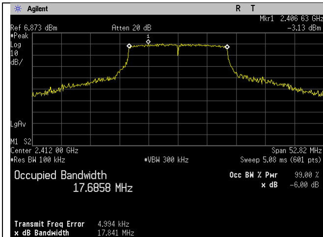
2412MHz_20MHz BW_n-mode_-6dB
