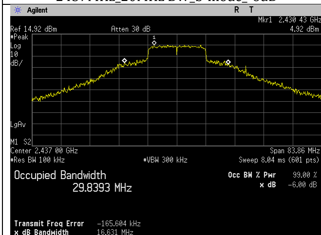
2437MHz_20MHz BW_g-mode_-6dB
