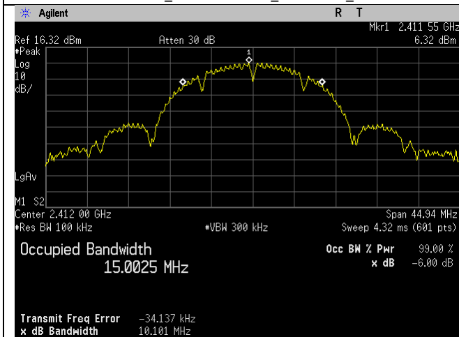
2412MHz_20MHz BW_b-mode_-6dB
