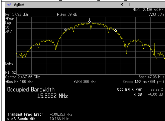
2437MHz_20MHz BW_b-mode_-6dB
