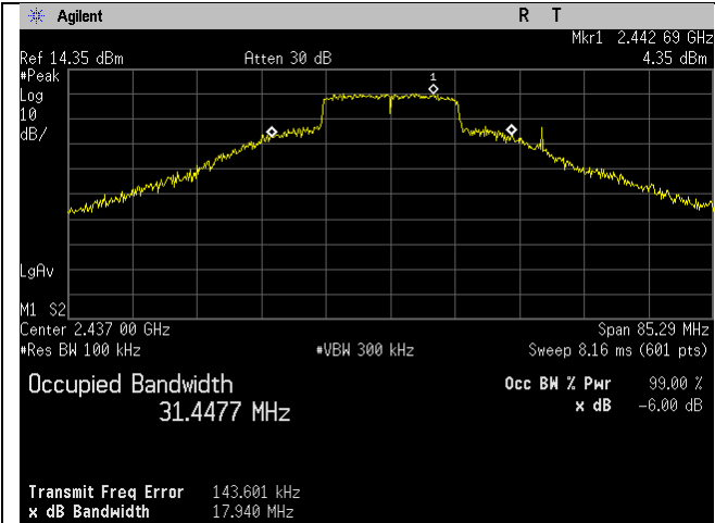
2437MHz_20MHz BW_n-mode_-6dB
