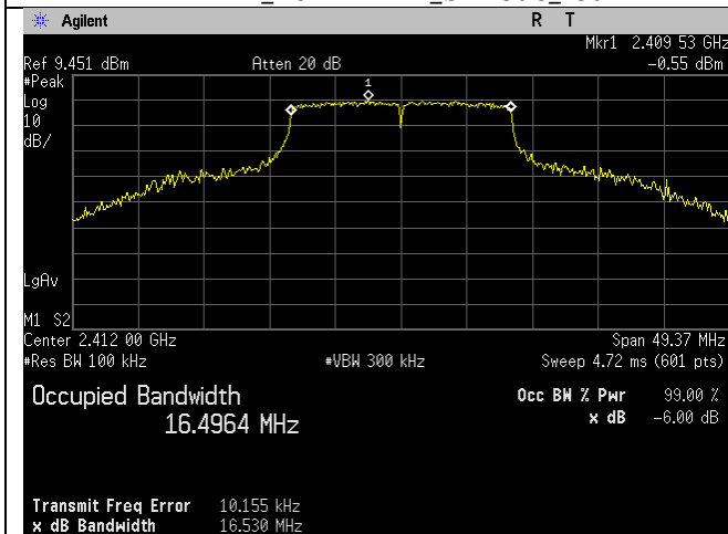
2412MHz_20MHz BW_g-mode_-6dB
