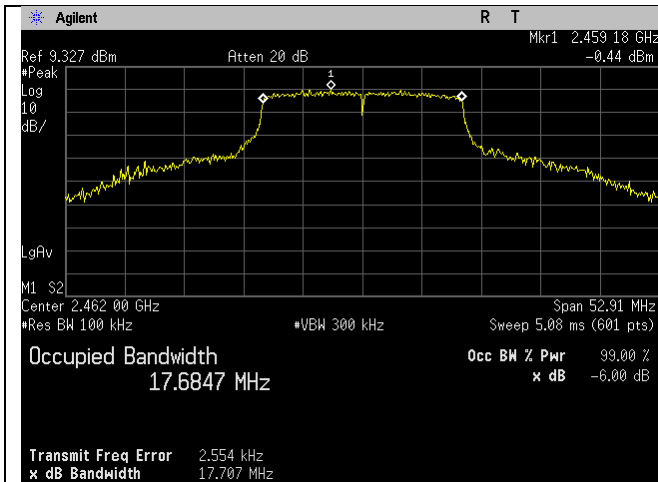
2462MHz_20MHz BW_n-mode_-6dB
