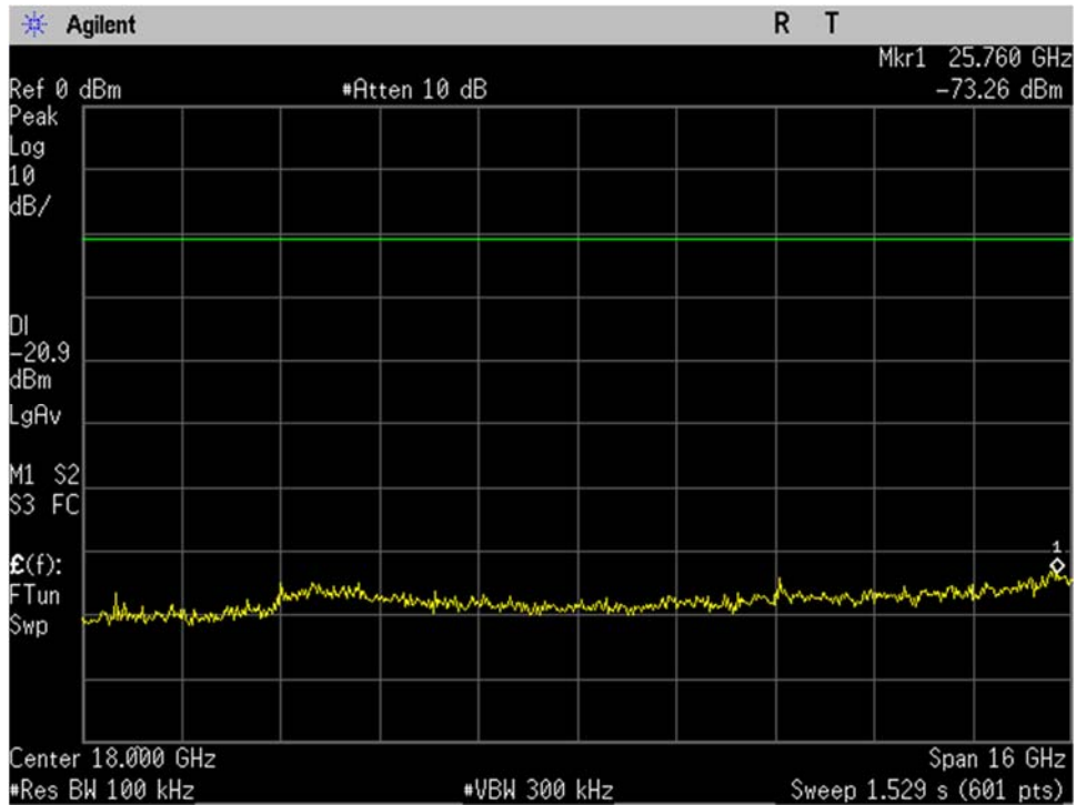
WIFI_Low Ch_2412MHz_20MHz BW_g-mode_-20dBc_10-26GHz_Port 2
