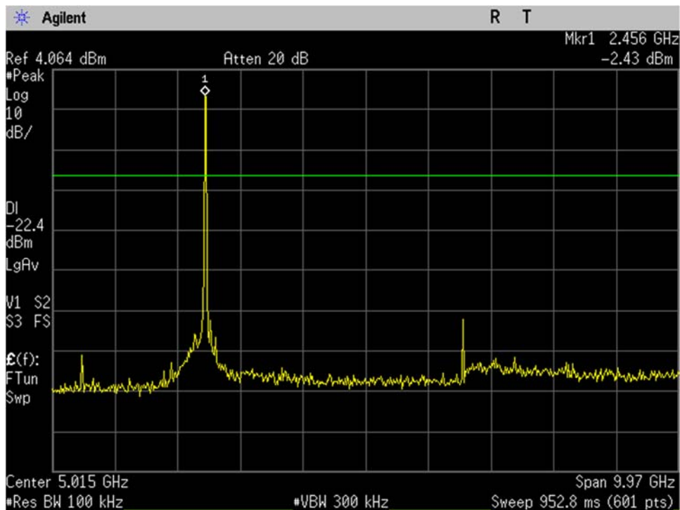
WIFI_High Ch_2462MHz_20MHz BW_n-mode_-20dBc_30MHz-10GHz_Port 1
