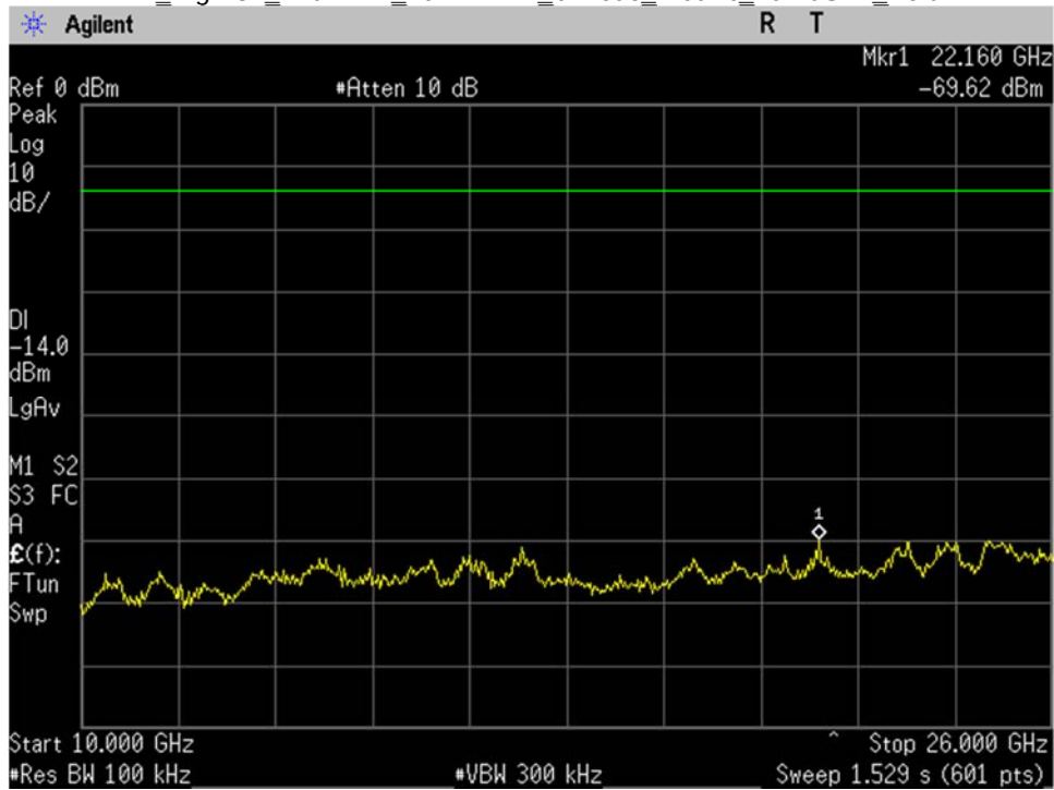
WIFI_High Ch_2462MHz_20MHz BW_b-mode_-20dBc_10-26GHz_Port 1
