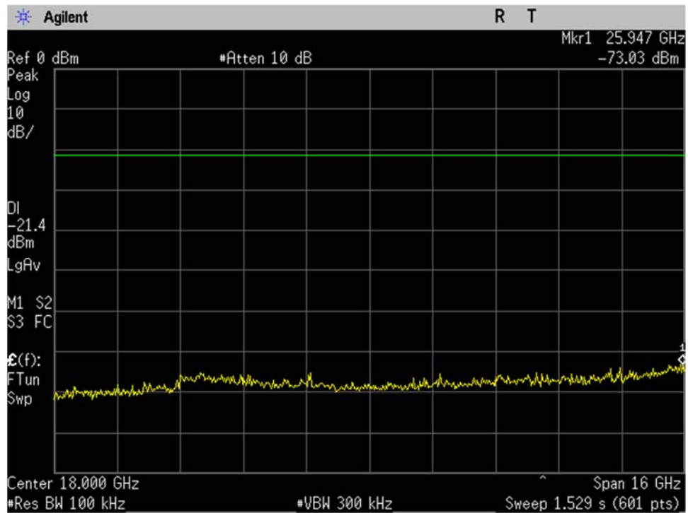
WIFI_Mid Ch_2437MHz_20MHz BW_g-mode_-20dBc_10-26GHz_Port 2
