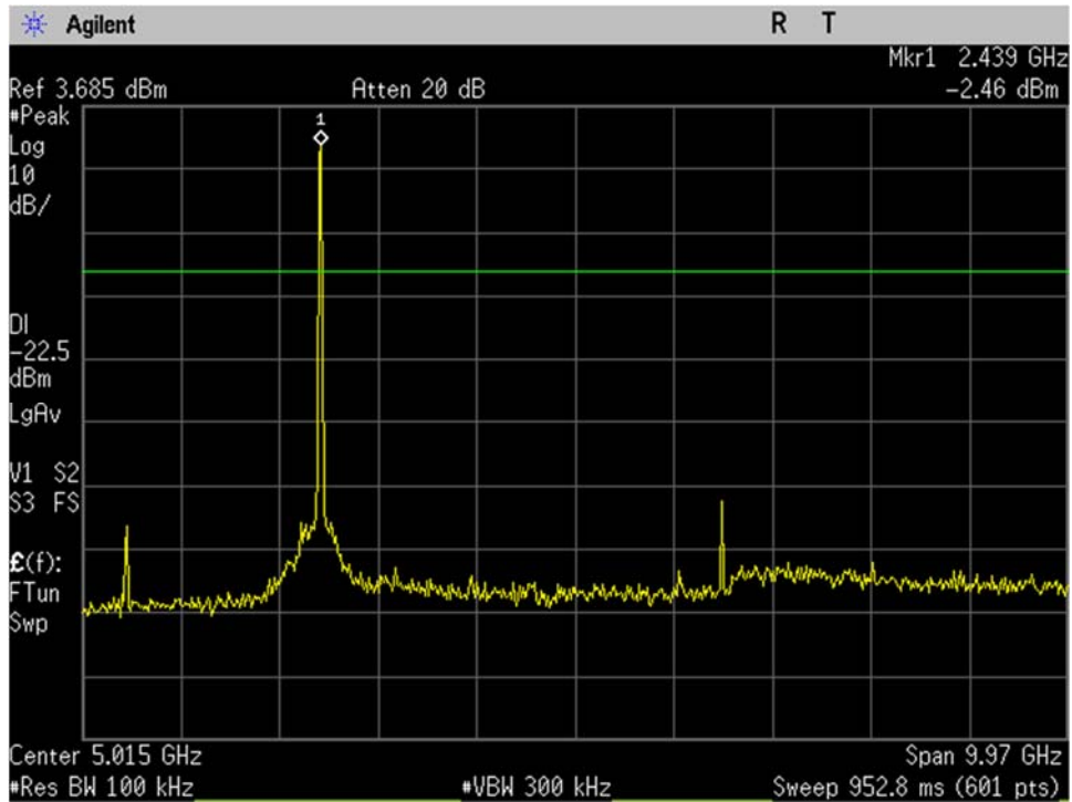
WIFI_Mid Ch_2437MHz_20MHz BW_n-mode_-20dBc_30MHz-10GHz_Port 1
