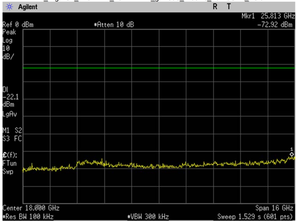
WIFI_High Ch_2462MHz_20MHz BW_g-mode_-20dBc_10-26GHz_Port 2
