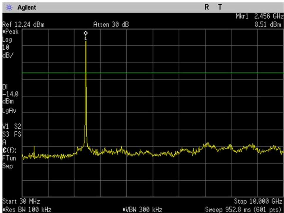
WIFI_High Ch_2462MHz_20MHz BW_b-mode_-20dBc_30MHz-10GHz_Port 1
