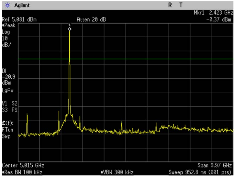
WIFI_Low Ch_2412MHz_20MHz BW_g-mode_-20dBc_30MHz-10GHz_Port 2
