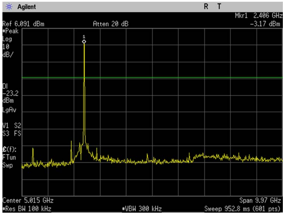
WIFI_Low Ch_2412MHz_20MHz BW_n-mode_-20dBc_30MHz-10GHz_Port 1
