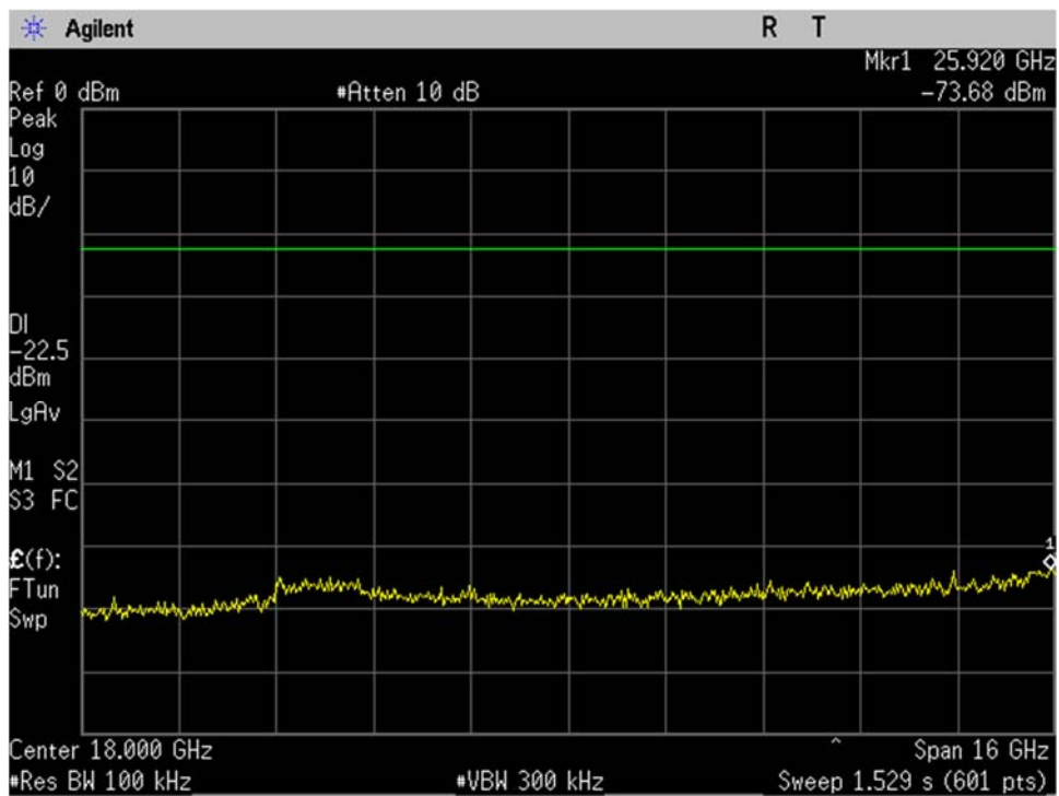
WIFI_Mid Ch_2437MHz_20MHz BW_n-mode_-20dBc_10-26GHz_Port 2
