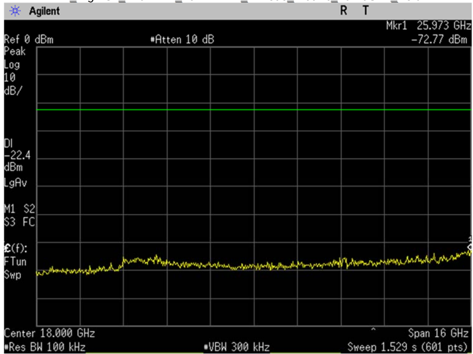
WIFI_High Ch_2462MHz_20MHz BW_n-mode_-20dBc_10-26GHz_Port 1
