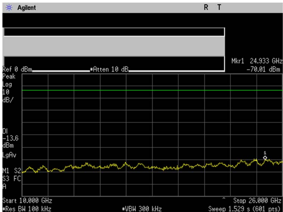
WIFI_Mid Ch_2437MHz_20MHz BW_b-mode_-20dBc_10-26GHz_Port 1
