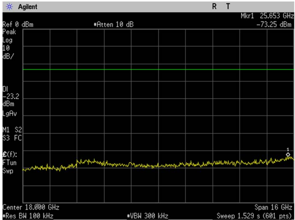
WIFI_Low Ch_2412MHz_20MHz BW_n-mode_-20dBc_10-26GHz_Port 2
