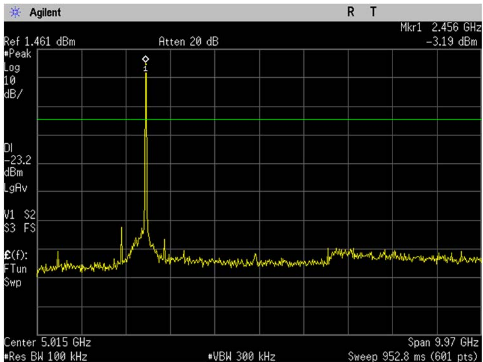
WIFI_High Ch_2462MHz_20MHz BW_n-mode_-20dBc_30MHz-10GHz_Port 2
