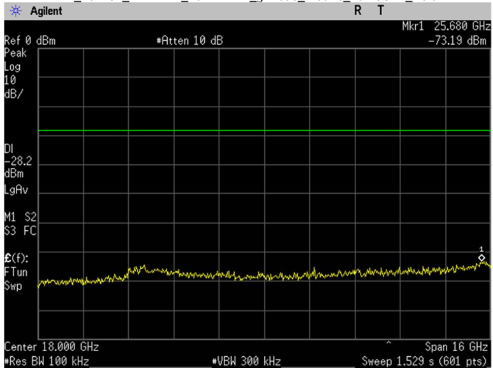
WIFI_Low Ch_2412MHz_20MHz BW_g-mode_-20dBc_10-26GHz_Port 1
