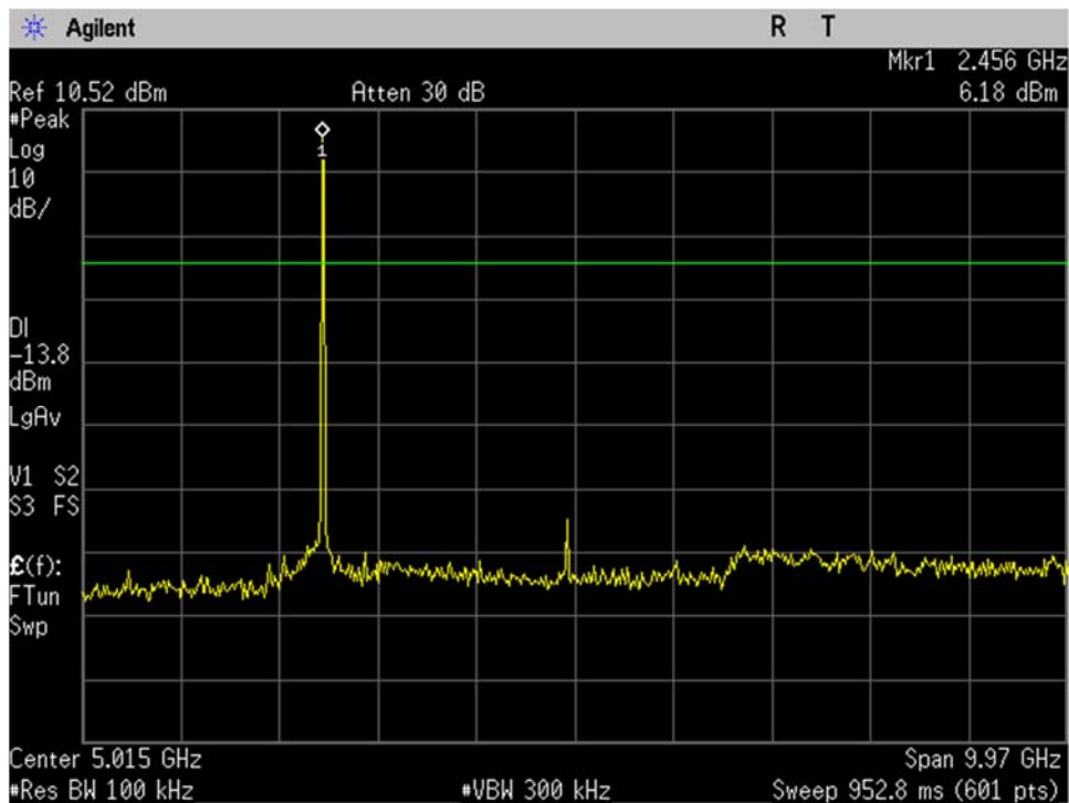
WIFI_High Ch_2462MHz_20MHz BW_b-mode_-20dBc_30MHz-10GHz_Port 2
