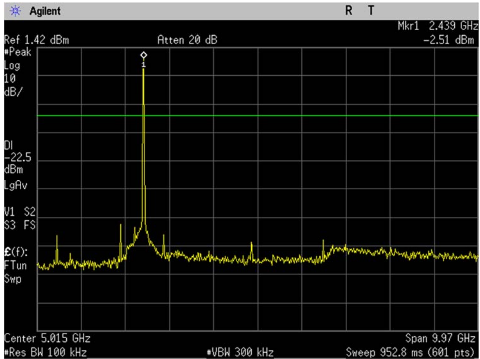
WIFI_Mid Ch_2437MHz_20MHz BW_n-mode_-20dBc_30MHz-10GHz_Port 2
