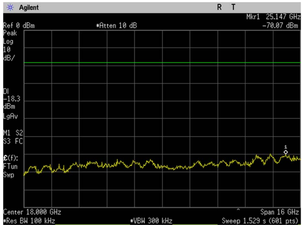
WIFI_High Ch_2462MHz_20MHz BW_g-mode_-20dBc_10-26GHz_Port 1
