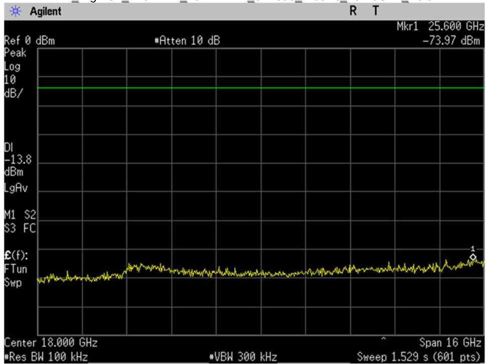
WIFI_High Ch_2462MHz_20MHz BW_b-mode_-20dBc_10-26GHz_Port 2
