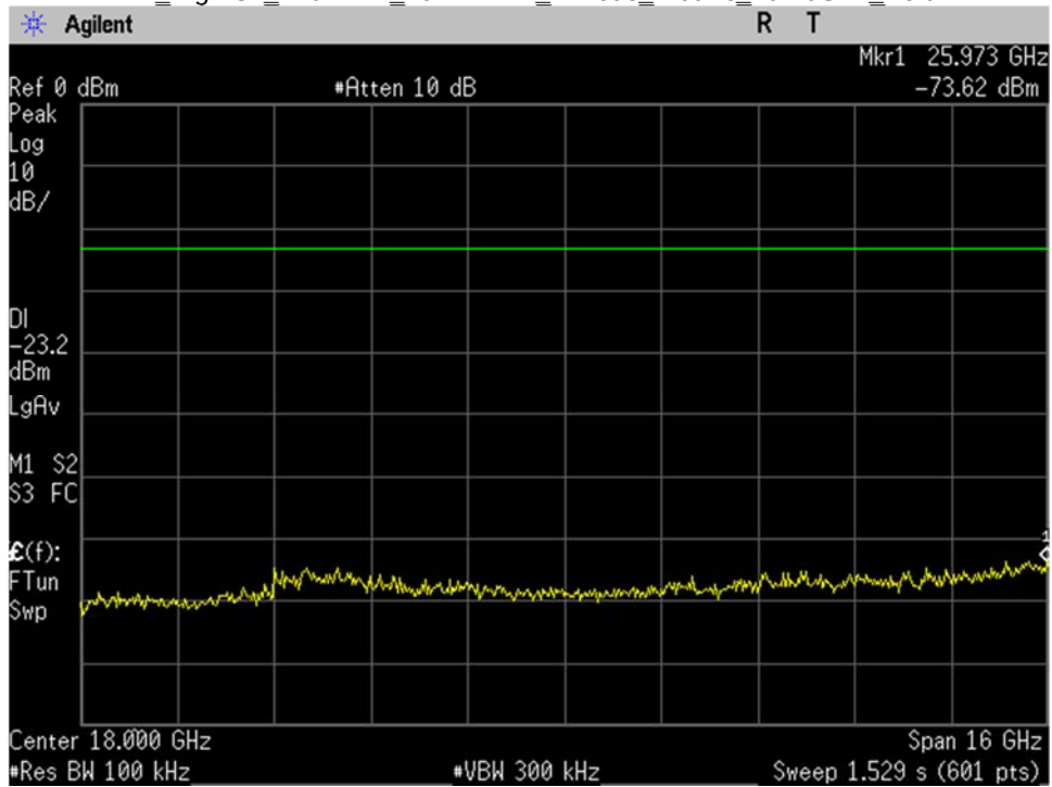
WIFI_High Ch_2462MHz_20MHz BW_n-mode_-20dBc_10-26GHz_Port 2
