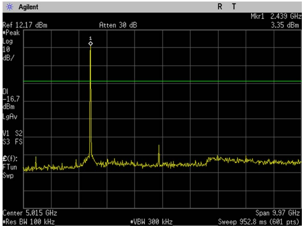
WIFI_Mid Ch_2437MHz_20MHz BW_b-mode_-20dBc_30MHz-10GHz_Port 2
