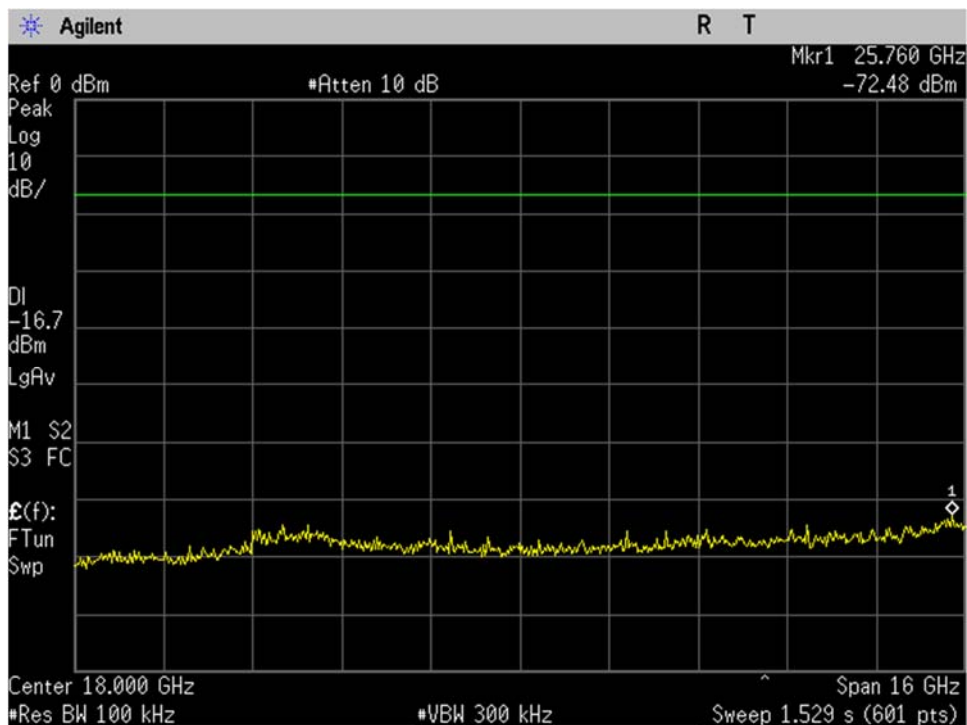
WIFI_Mid Ch_2437MHz_20MHz BW_b-mode_-20dBc_10-26GHz_Port 2
