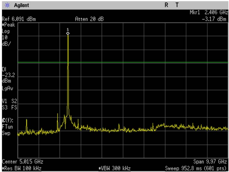
WIFI_Low Ch_2412MHz_20MHz BW_n-mode_-20dBc_30MHz-10GHz_Port 2
