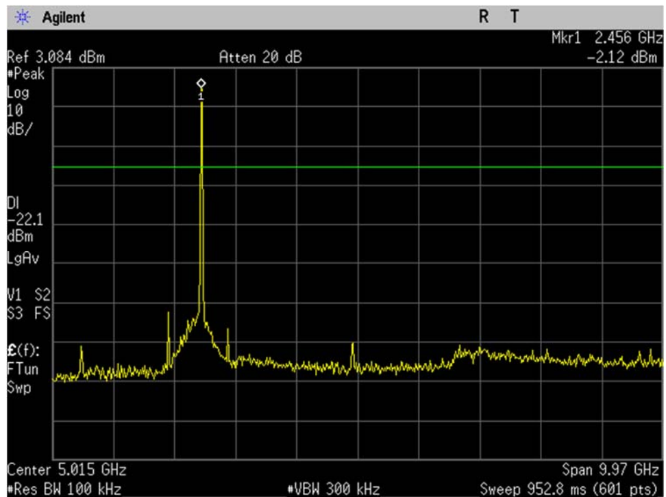
WIFI_High Ch_2462MHz_20MHz BW_g-mode_-20dBc_30MHz-10GHz_Port 2
