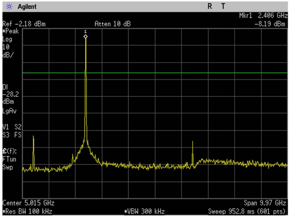
WIFI_Low Ch_2412MHz_20MHz BW_g-mode_-20dBc_30MHz-10GHz_Port 1
