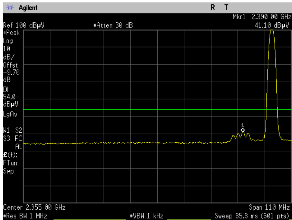
Low Ch_2402MHz_Pi_4DQPSK_15.209_Lower Band Edge Avg_Port 1
