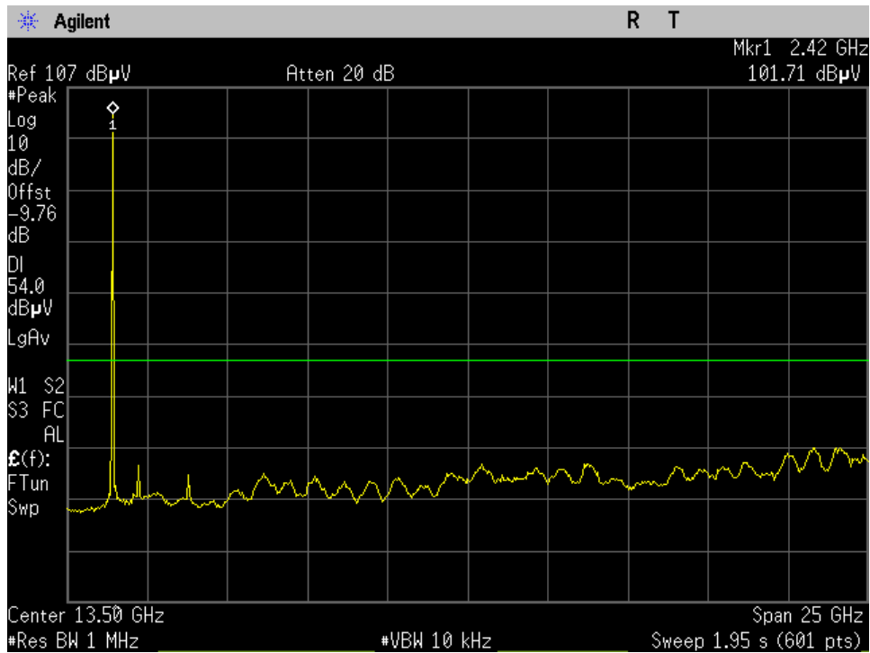
Low Ch_2402MHz_Pi_4DQPSK_15.209_1-26GHz avg_Port 1
