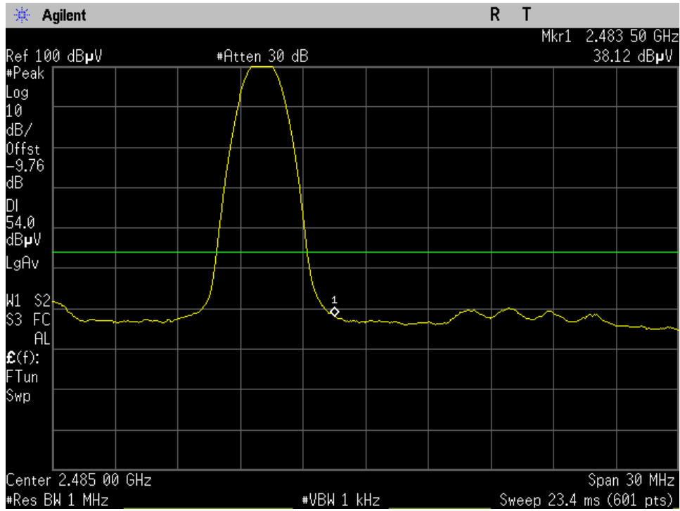
High Ch_2480MHz_Pi_4DQPSK_15.209_Upper Band Edge Avg_Port 1
