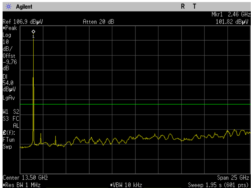
Mid Ch_2440MHz_Pi_4DQPSK_15.209_1-26GHz avg_Port 1
