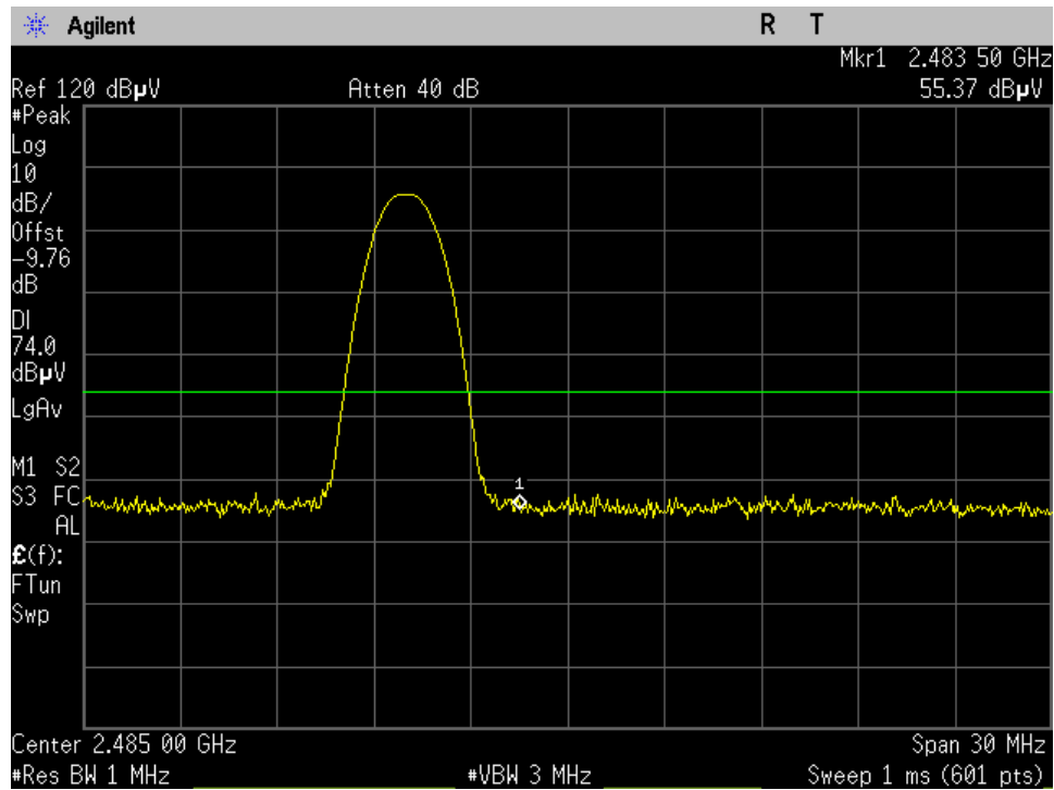
High Ch_2480MHz_Pi_4DQPSK_15.209_Upper Band Edge Peak_Port 1
