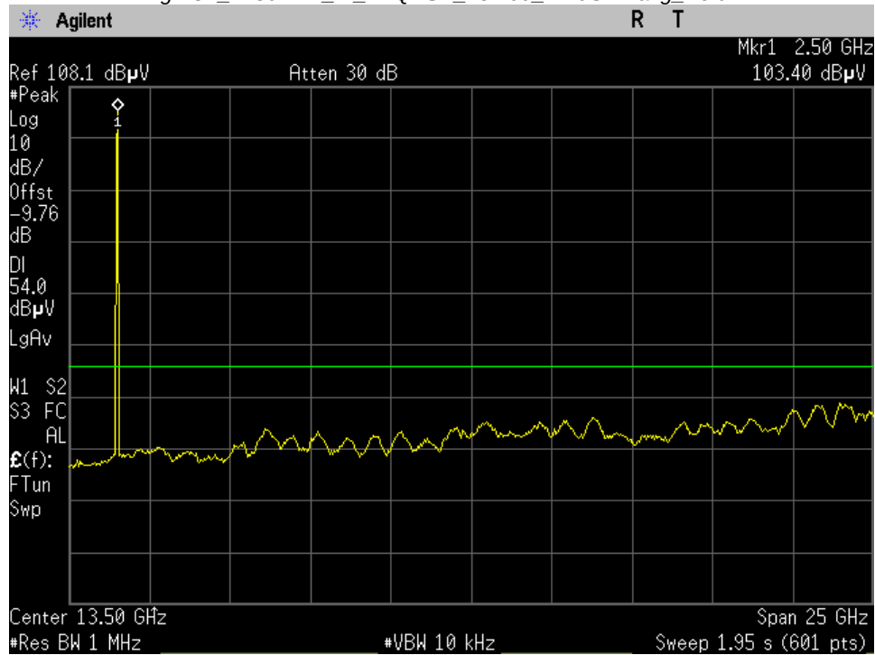
High Ch_2480MHz_Pi_4DQPSK_15.209_1-26GHz avg_Port 1
