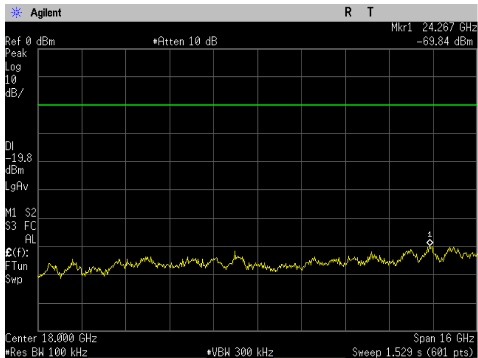
Mid Ch_2440MHz_Pi_4DQPSK_-20dBc_10-26GHz_Port 1
