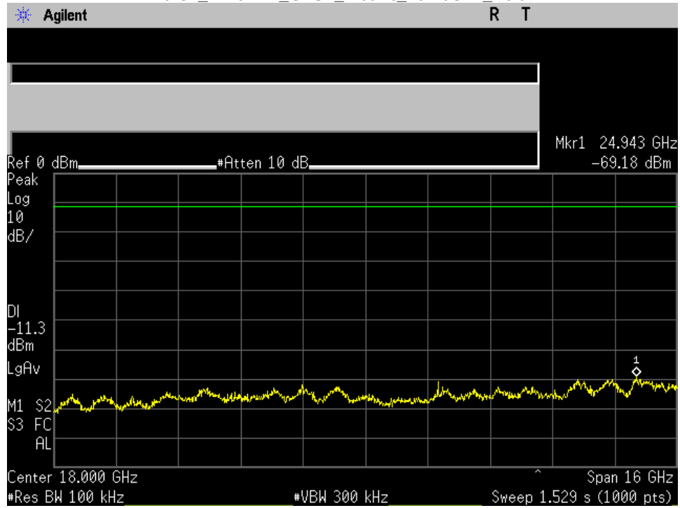
Mid Ch_2440MHz_GFSK_-20dBc_10-26GHz_Port 1
