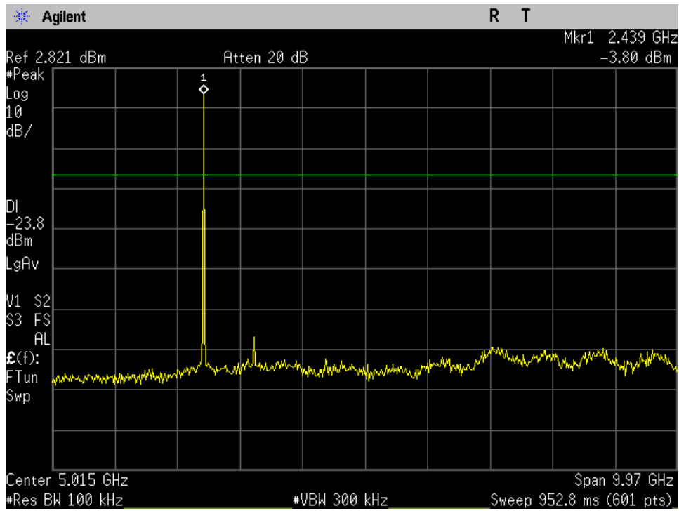
Mid Ch_2440MHz_8DPSK_-20dBc_30MHz-10GHz_Port 1
