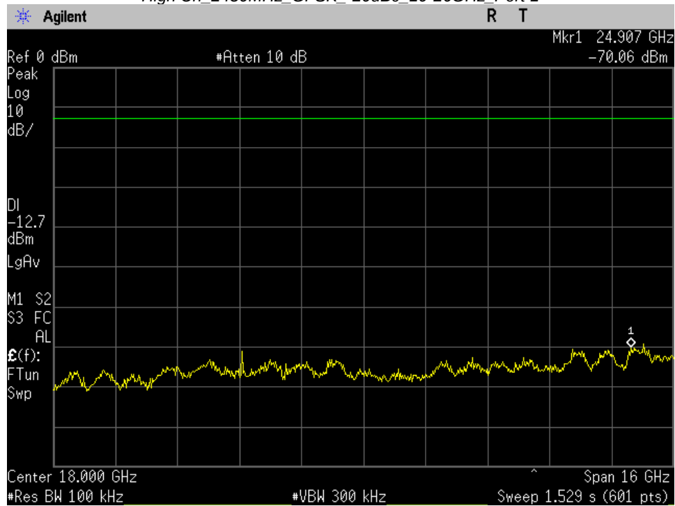
High Ch_2480MHz_GFSK_-20dBc_10-26GHz_Port 1
