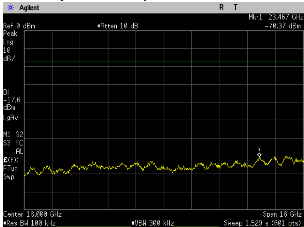
High Ch_2480MHz_Pi_4DQPSK_-20dBc_10-26GHz_Port 1
