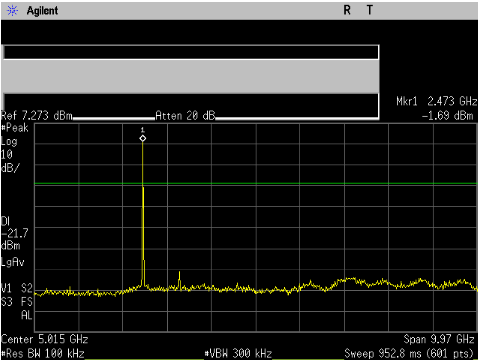
High Ch_2480MHz_8DPSK_-20dBc_30MHz-10GHz_Port 1
