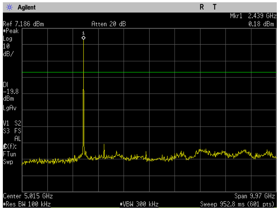
Mid Ch_2440MHz_Pi_4DQPSK_-20dBc_30MHz-10GHz_Port 1
