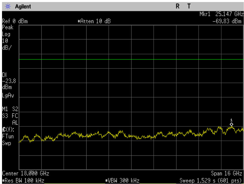
Mid Ch_2440MHz_8DPSK_-20dBc_10-26GHz_Port 1
