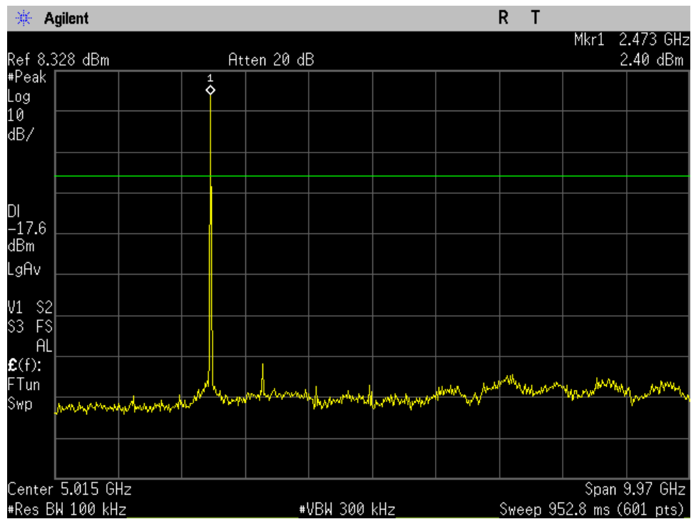
High Ch_2480MHz_Pi_4DQPSK_-20dBc_30MHz-10GHz_Port 1
