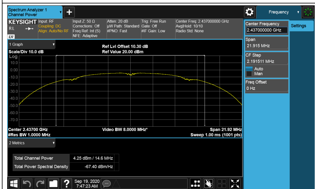
802.11b-2437MHz
