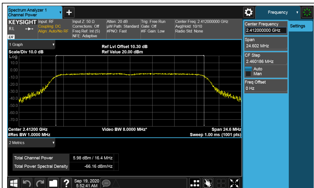
802.11g-2412MHz
