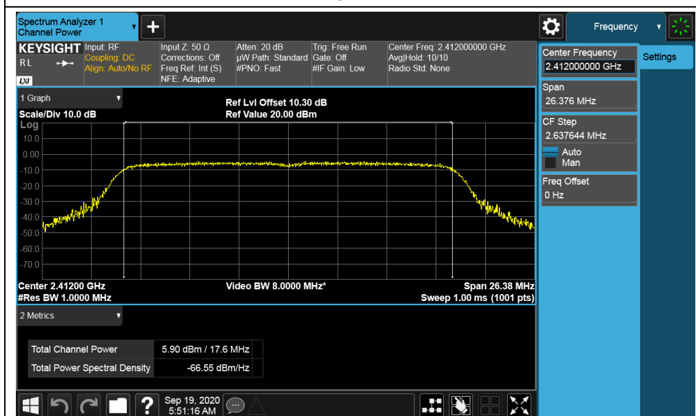
802.11n-HT20-2412MHz
