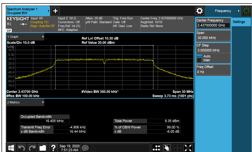
802.11g-2437MHz
