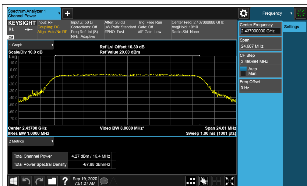
802.11g-2437MHz
