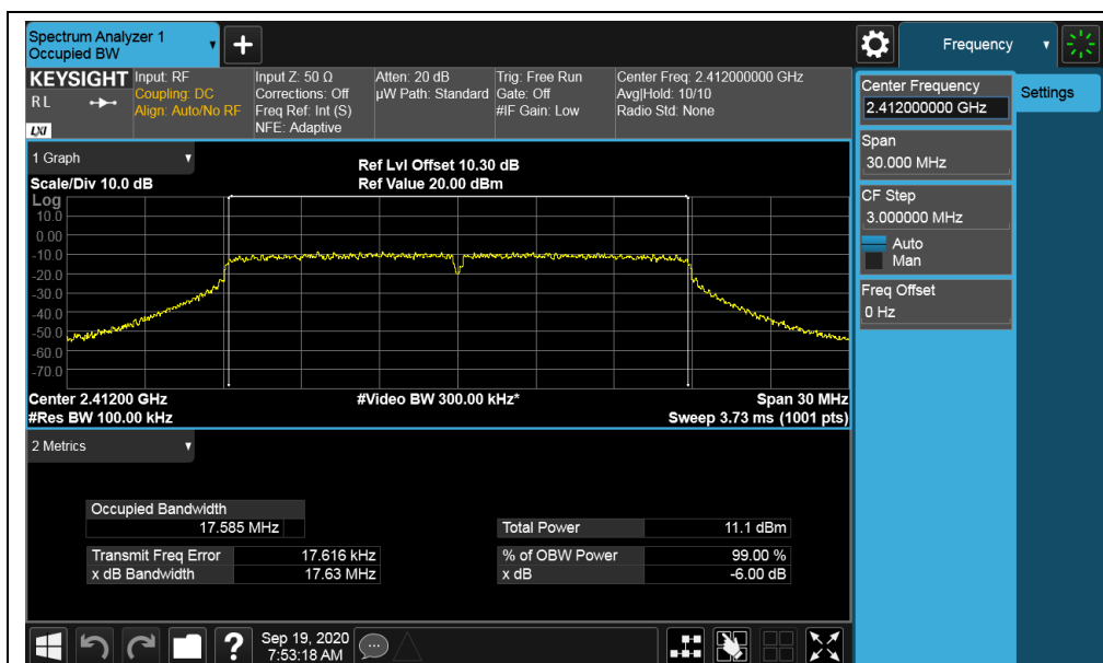
802.11n-HT20-2412MHz
