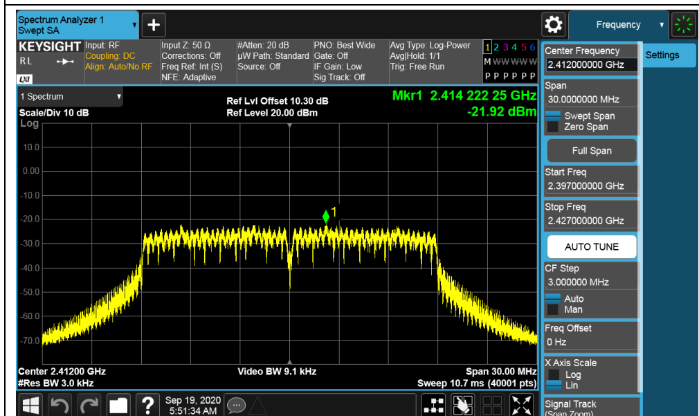
802.11n-HT20-2412MHz
