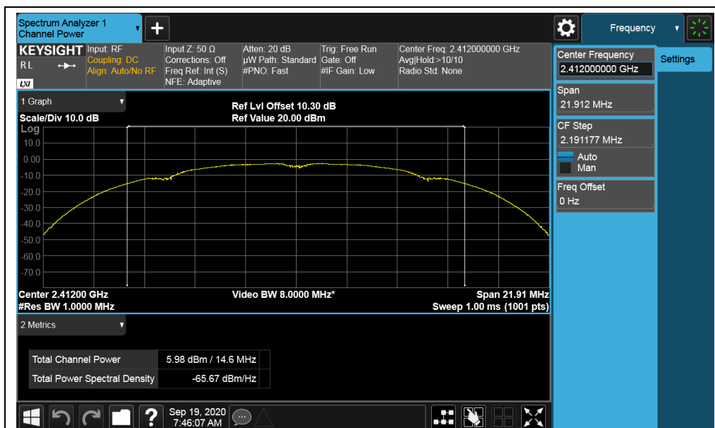
802.11b-2412MHz
