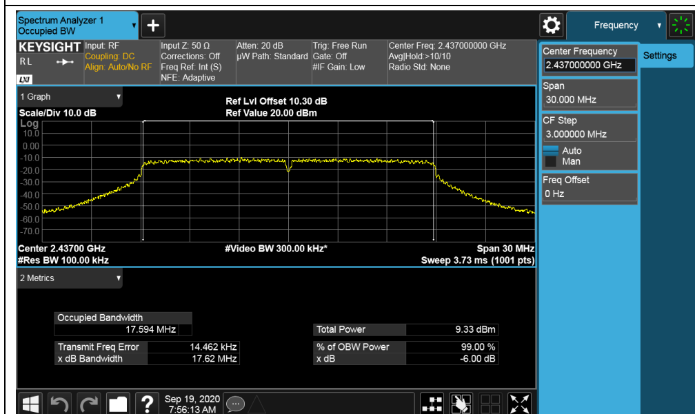
802.11n-HT20-2437MHz
