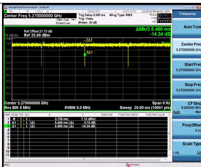
11AX40MIMO_Ant6_5270
