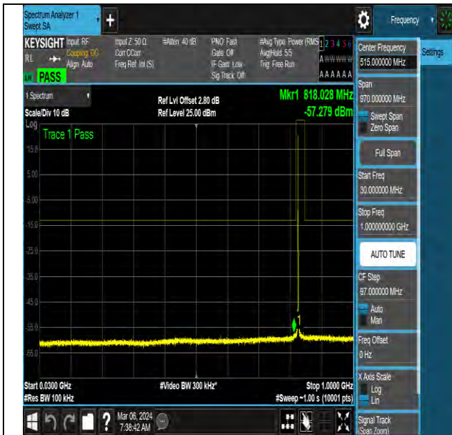
NTNV-N5-PC3-15-20-H-DFT-QPSK-Edge_1RB_Left-Ant0-P ASS
