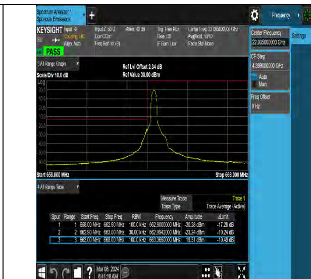
NTNV-N71-PC3-15-5-L-DFT-QPSK-Edge_1RB_Left-Ant0-PA SS
