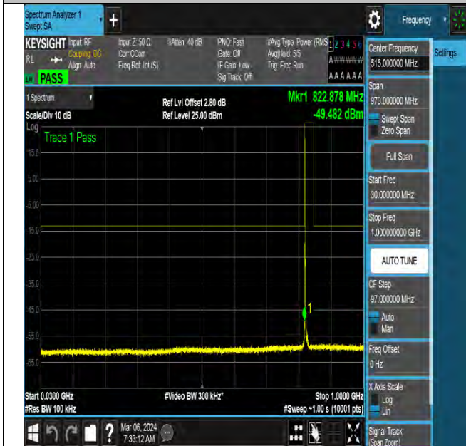
NTNV-N5-PC3-15-10-L-DFT-QPSK-Edge_1RB_Left-Ant0-PA SS
