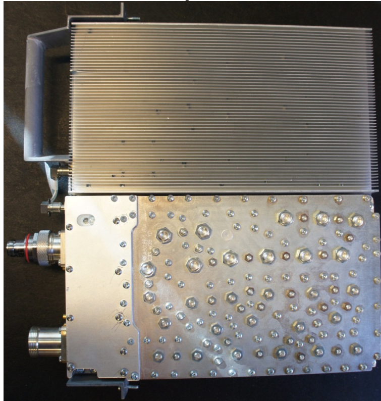
Top side
