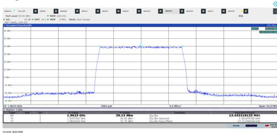
Diagram 1.5, E-TM1.1, M 15 , Port A:
