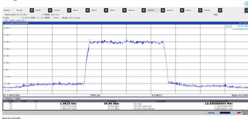
Diagram 1.13, E-TM3.2, M 15 , Port A:
