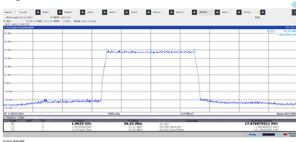
Diagram 1.6, E-TM1.1, M 20 , Port A:
