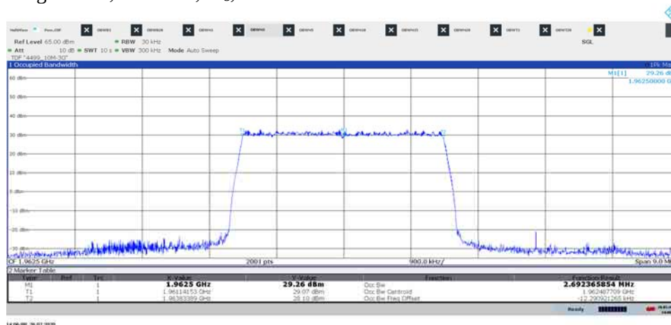
Diagram 1.2, E-TM1.1, M_3 , Port A:
