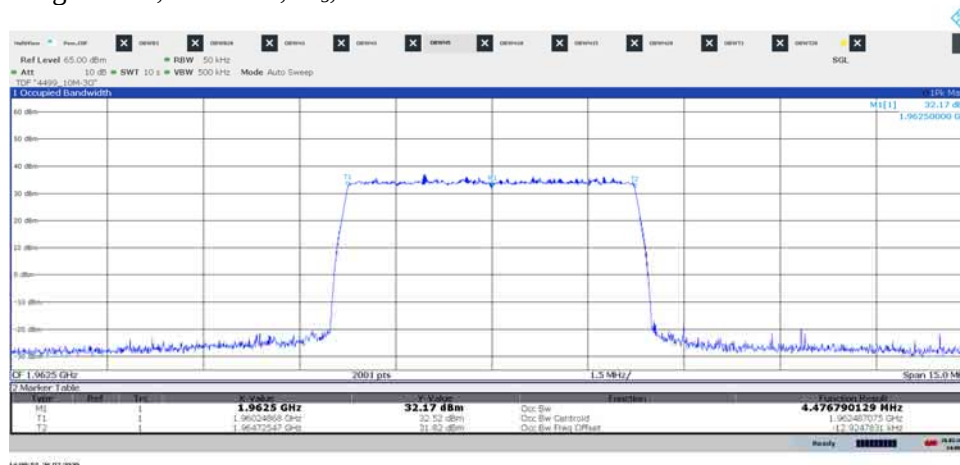
Diagram 1.3, E-TM1.1, M_5 , Port A:
