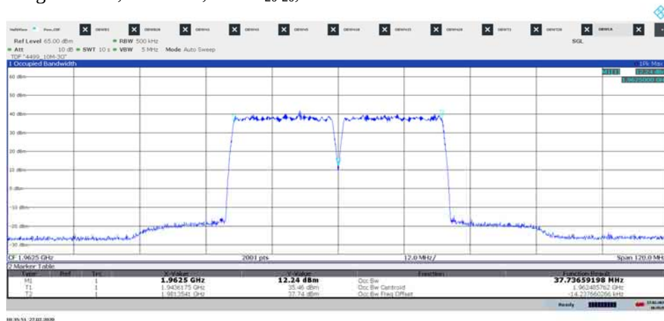
Diagram 1.15, E-TM3.2, CA-M 20-20 , Port A:
