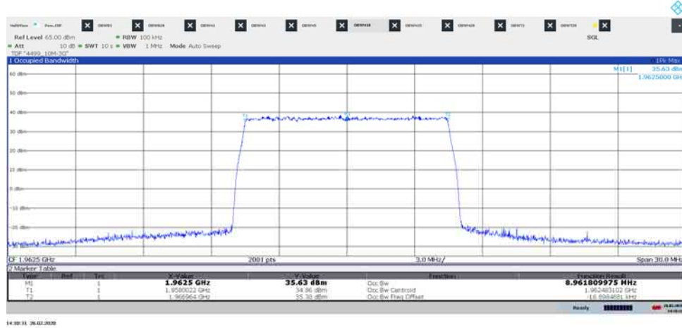
Diagram 1.4, E-TM1.1, M 10 , Port A:
