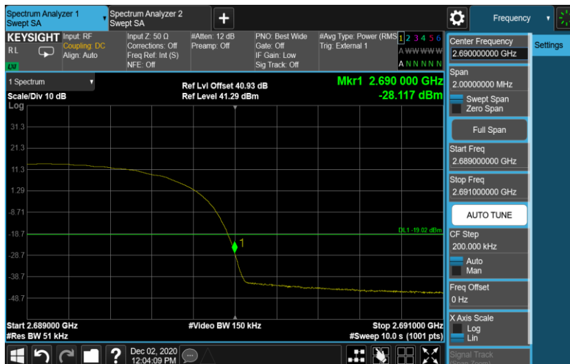
Port D, Channel Position T, WCDMA 5.0MHz, NR 20.0MHz
