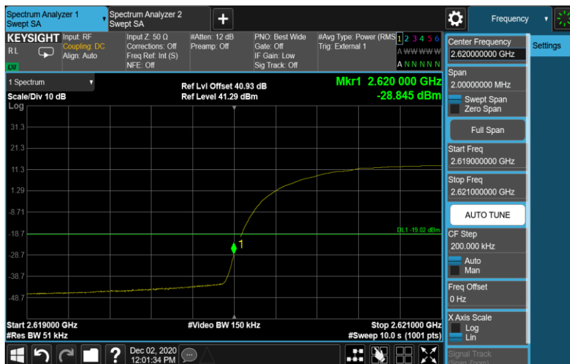
Port D, Channel Position B, WCDMA 5.0MHz, NR 20.0MHz
