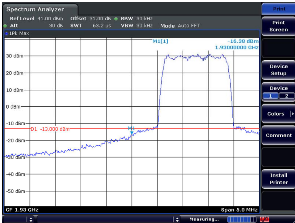
Band Edge (ch25)
