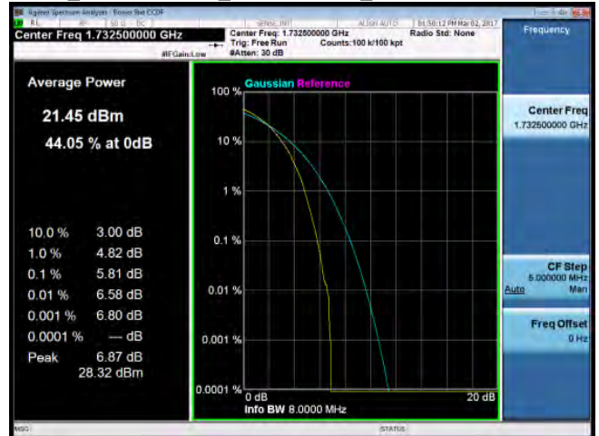
LTE_Band4 10MHz_16-QAM 50 0_MidCH20175-1732.5
