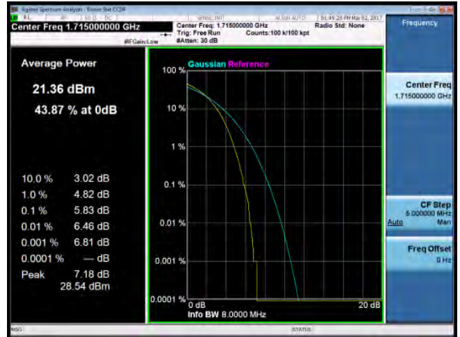
LTE_Band4 10MHz_16-QAM 50 0_LowCH20000-1715
