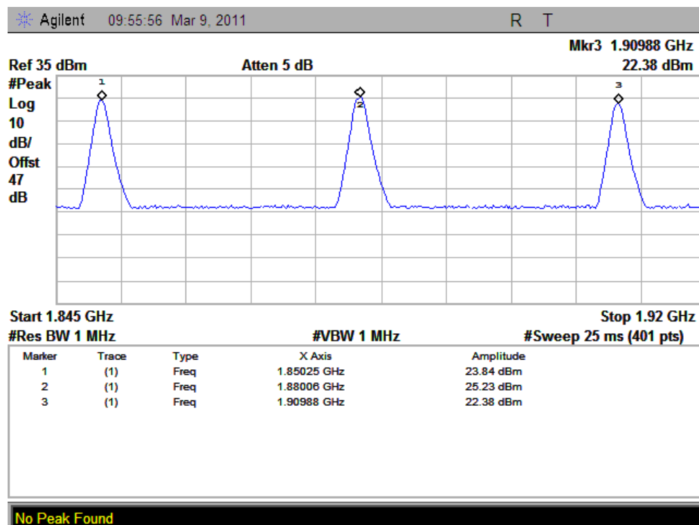
(Plot J: EDGE 1900MHz Channel = 512, 661, 810)
