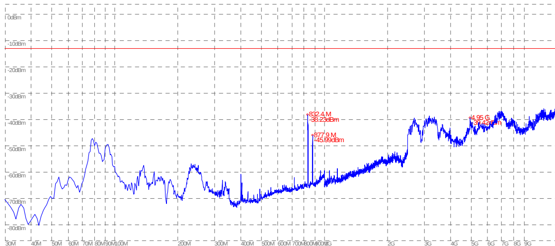
(Plot N.1: WCDMA 850MHz Channel = 4175, Test Antenna Horizontal)
