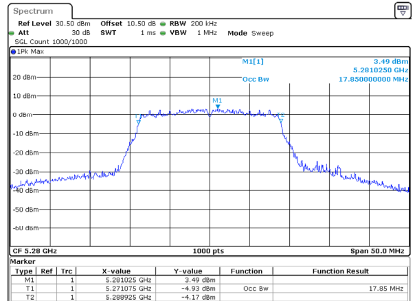
802.11ac20_5280MHz
