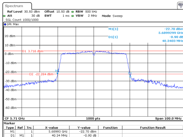
802.11ac40_5710MHz
