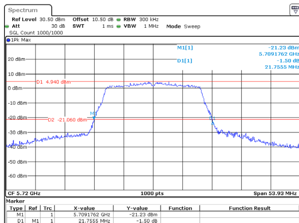
802.11ac20_5720MHz
