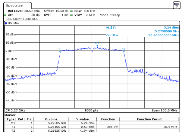
802.11ac40_5270MHz
