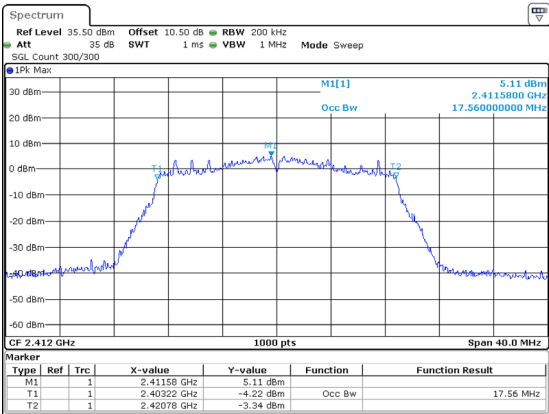
802.11n20_2412MHz
