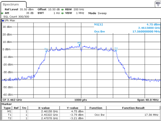
802.11n20_2462MHz
