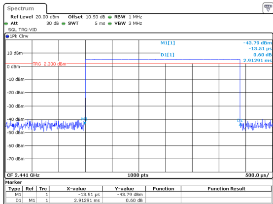
DH5_Hopping 2.913ms
