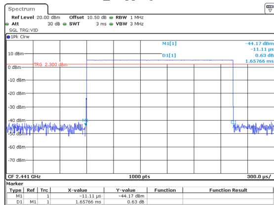
DH3_Hopping 1.658ms
