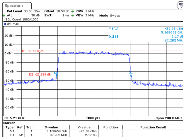
802.11ax80_5210MHz_RU_Full
