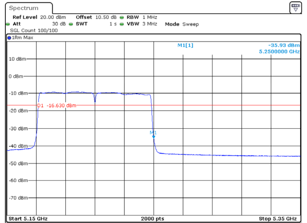
802.11ac80_5210MHz
