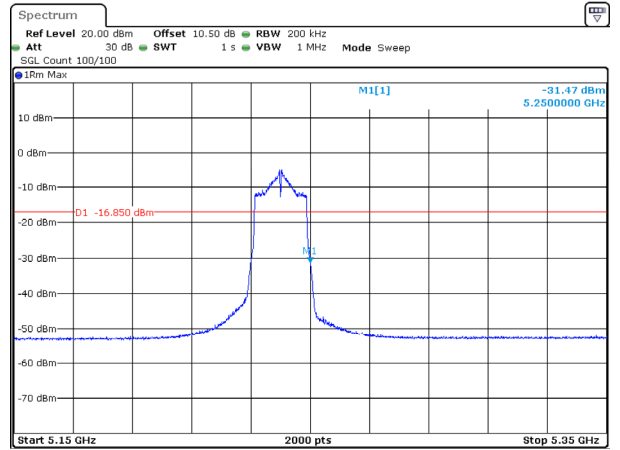
802.11ac20_5240MHz
