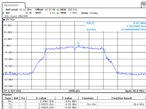
802.11g_2437MHz
