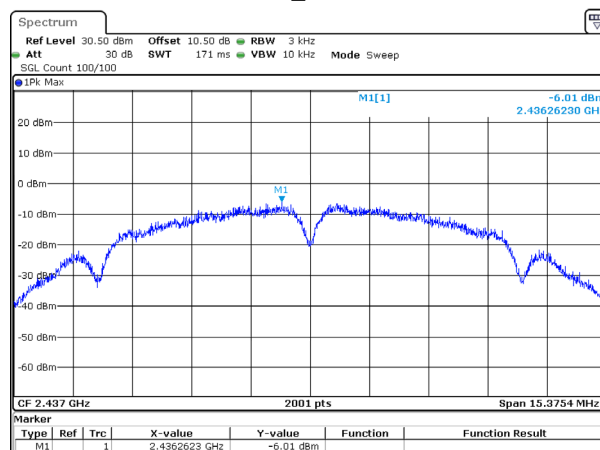
802.11b_2437MHz
