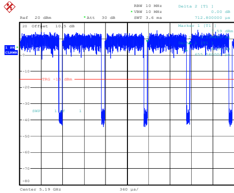
802.11ac40_5190MHz
