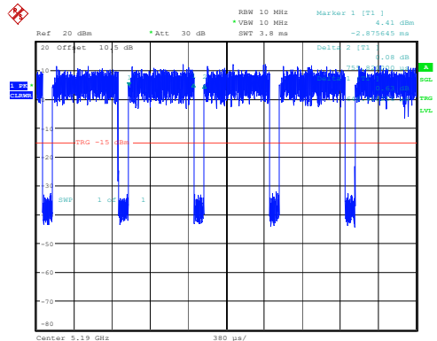
802.11ac40_5190MHz_Chain 1
