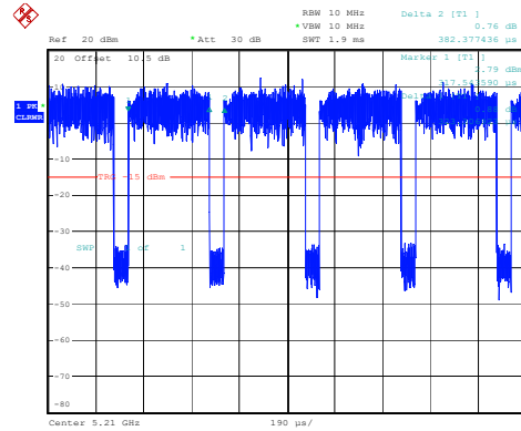
802.11ac80_5210MHz
