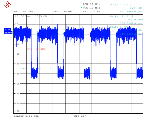
802.11ac80_5210MHz_Chain 1
