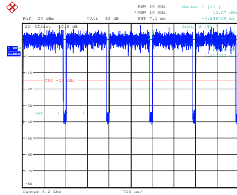
802.11ac20_5200MHz_Chain 1
