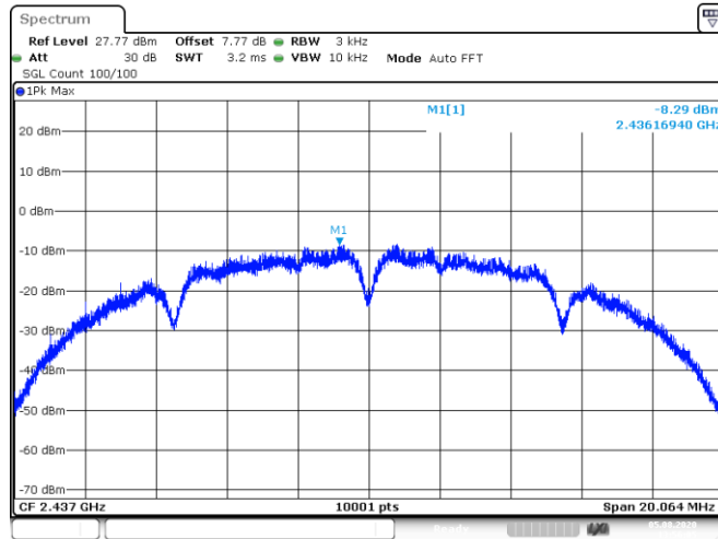
PSD NVNT 802.11b 2437MHz Ant1
