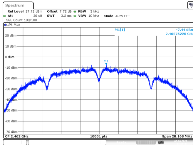
PSD NVNT 802.11b 2462MHz Ant1
