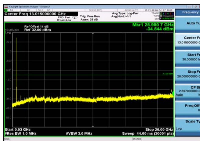
FDD17_HighRange_5MHz_30MHz~26GHz
