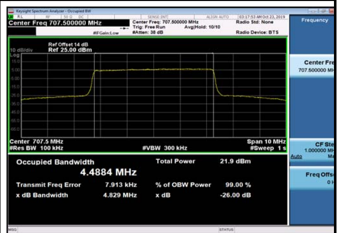
FDD12_MidRange_10_707.5_Q16
