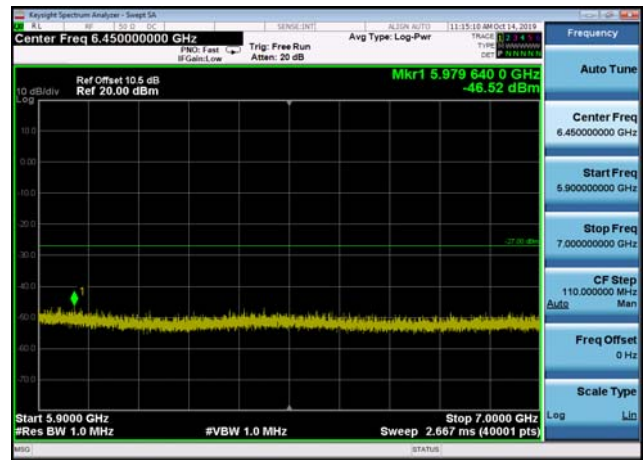
U-NII-3 ,Plot 3,5900MHz~7000MHz-802.1 1n(40MHz),5795MHz,Ant2
