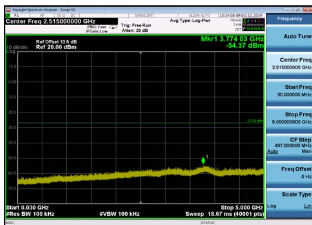
U-NII-2c ,Plot 2,30MHz~5000MHz-802.11 ac(20MHz),5700MHz,Ant2
