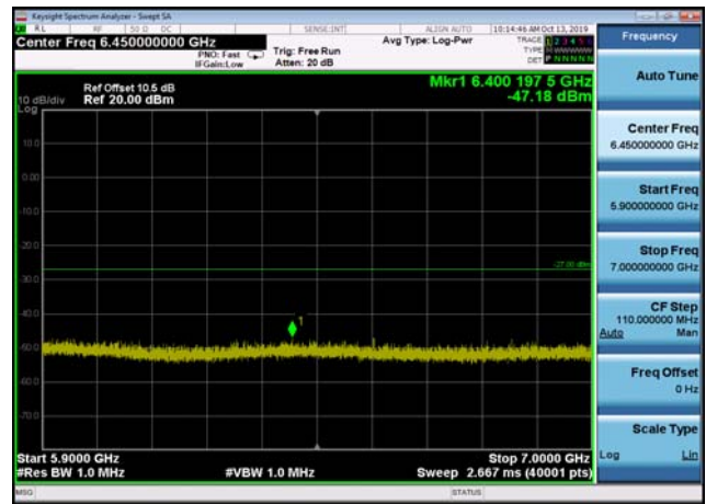
U-NII-2c ,Plot 3,5900MHz~7000MHz-802. 11ac(20MHz),5700MHz,Ant2
