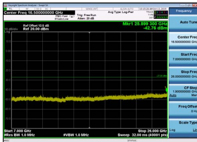
U-NII-2c ,Plot 4,7000MHz~26000MHz-802 .11ac(20MHz),5700MHz,Ant2
