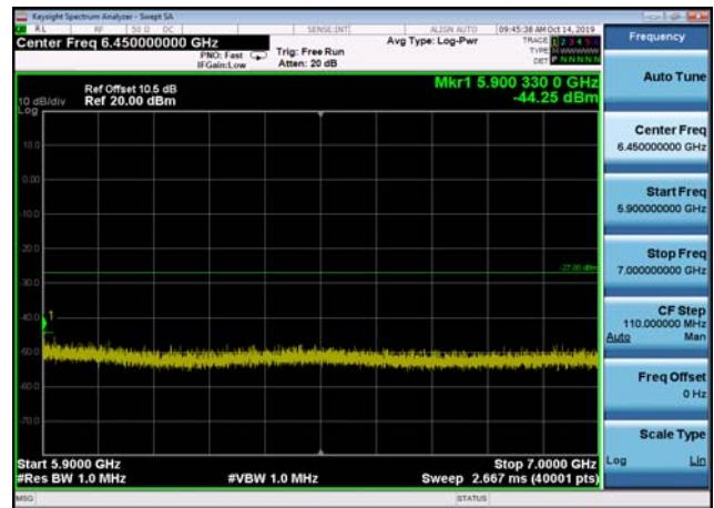
U-NII-3 ,Plot 3,5900MHz~7000MHz-802.1 1n(20MHz),5825MHz,Ant2
