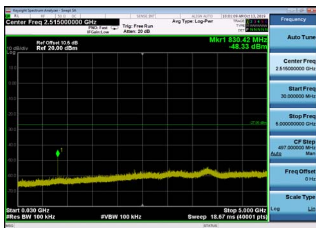
U-NII-2c ,Plot 2,30MHz~5000MHz-802.11 ac(40MHz),5510MHz,Ant2
