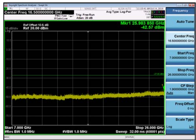
U-NII-3 ,Plot 4,7000MHz~26000MHz-802. 11n(40MHz),5755MHz,Ant2
