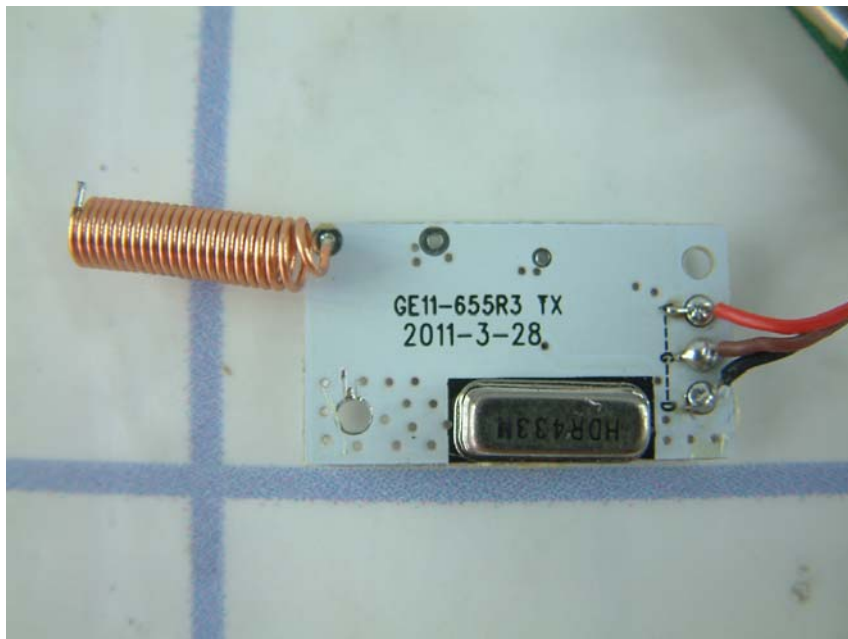
RF Module view-1
