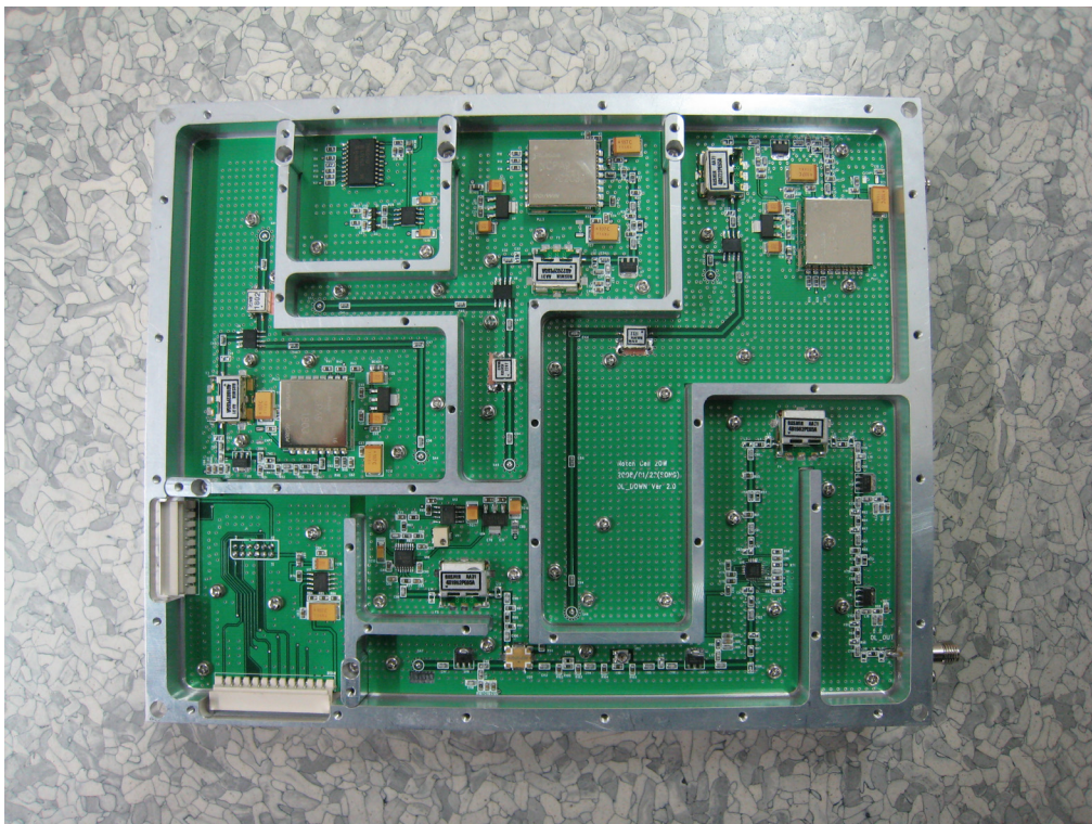
<UL UDC BOTTOM View>
