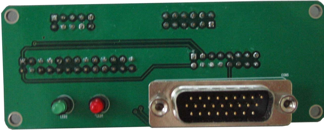
<BOTTOM SIDE>
