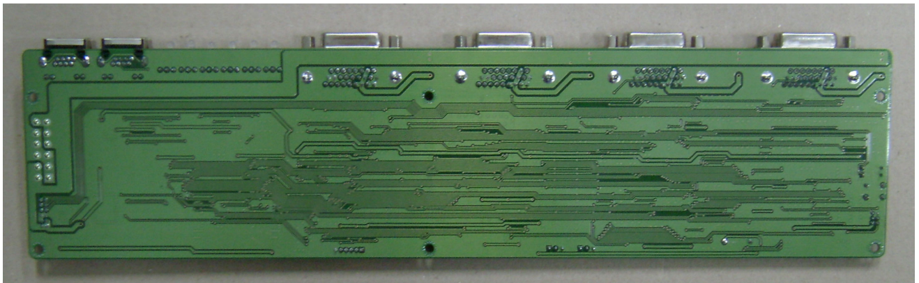
<BOTTOM SIDE>
