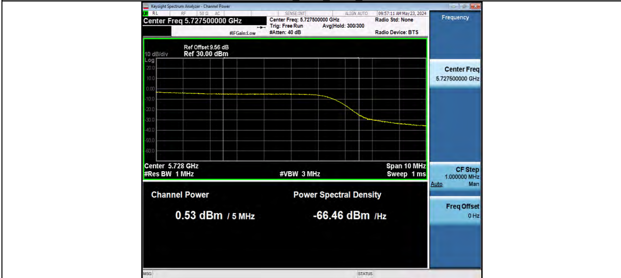
11N20MIMO Ant1 5745
