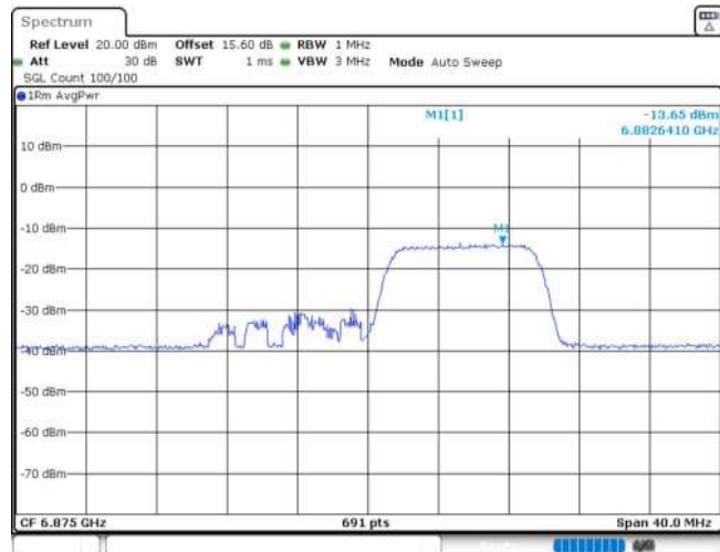
11AX20MIMO_Ant2_6875_106Tone_RU54
