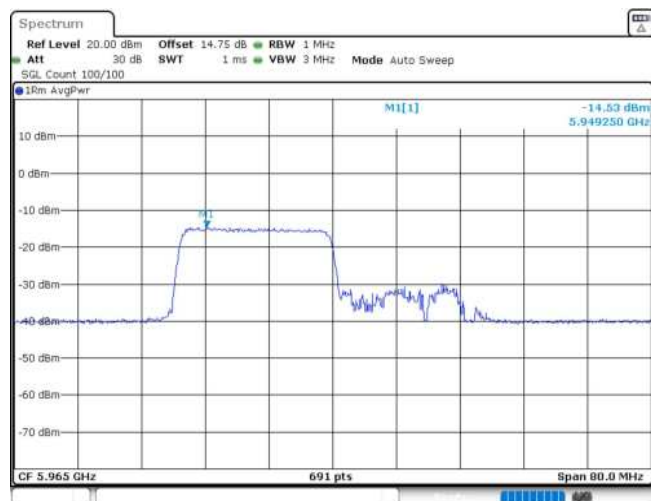
11AX40MIMO_Ant1_5965_242Tone_RU61
