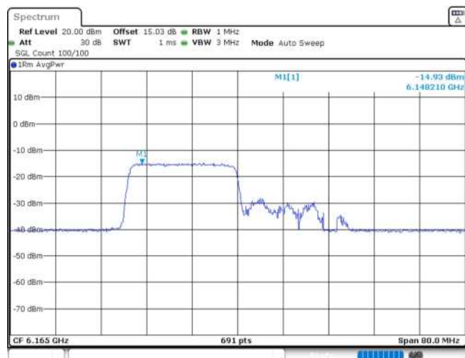
11AX40MIMO_Ant2_6165_242Tone_RU61
