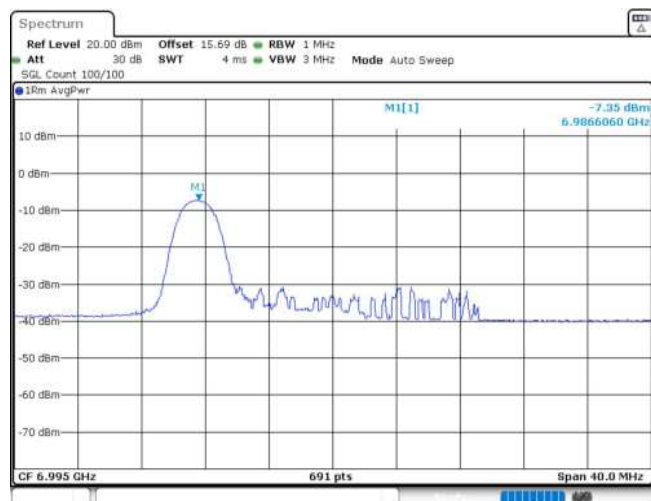
11AX20MIMO_Ant2_6995_26Tone_RU0
