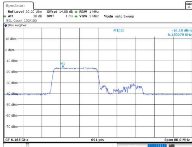
11AX40MIMO_Ant1_6165_242Tone_RU61
