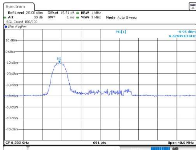
11AX20MIMO_Ant1_6535_106Tone_RU54
