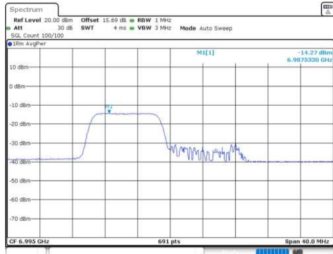
11AX20MIMO_Ant2_6995_106Tone_RU53
