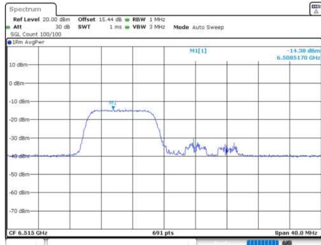
11AX20MIMO_Ant1_6515_106Tone_RU53
