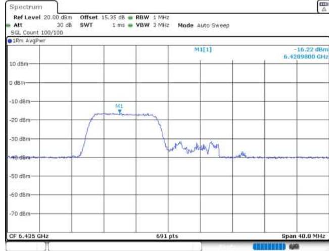
11AX20MIMO_Ant2_6435_106Tone_RU53
