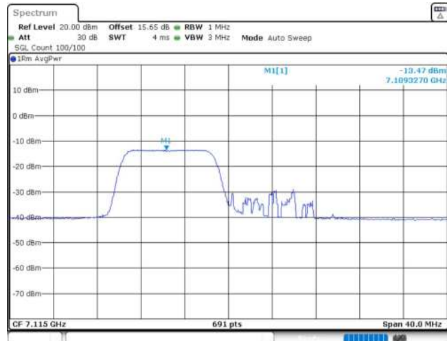
11AX20MIMO_Ant2_7115_106Tone_RU53
