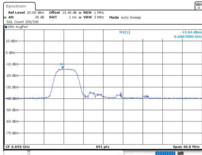
11AX20MIMO_Ant2_6695_52Tone_RU37
