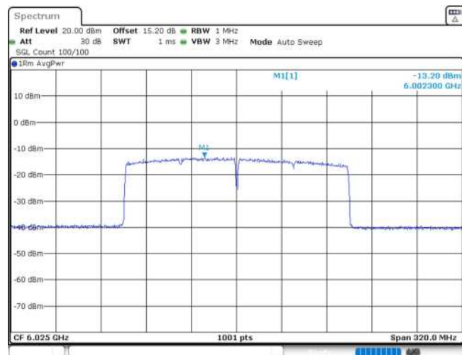
11AX160MIMO_Ant1_6025
