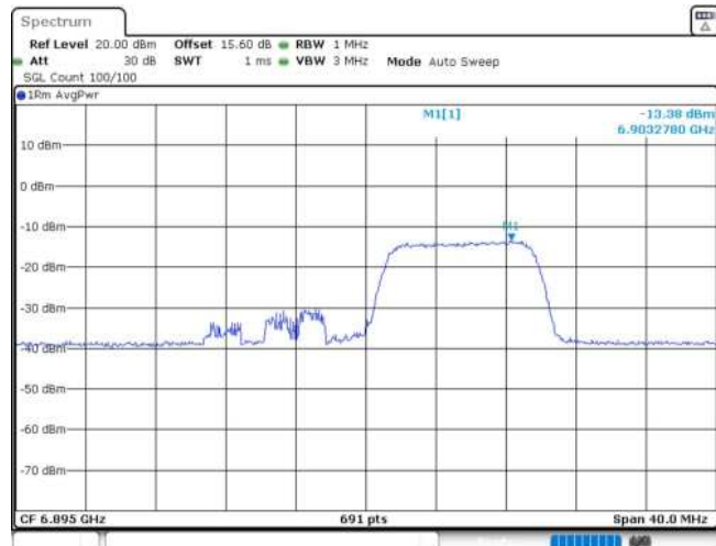
11AX20MIMO_Ant2_6895_106Tone_RU54
