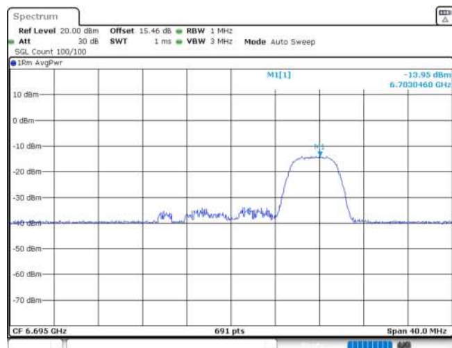
11AX20MIMO_Ant2_6695_52Tone_RU40
