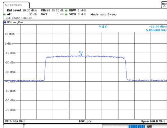
11AX80MIMO_Ant2_6865
