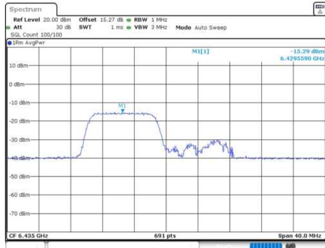
11AX20MIMO_Ant1_6435_106Tone_RU53
