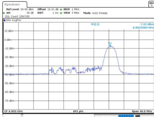
11AX20MIMO_Ant1_6855_26Tone_RU8
