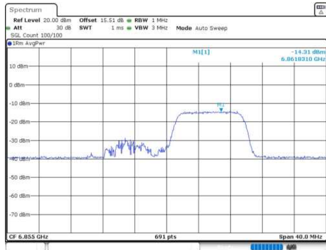
11AX20MIMO_Ant1_6855_106Tone_RU54
