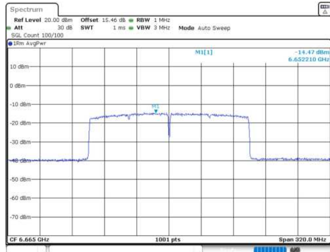
11AX160MIMO_Ant2_6665
