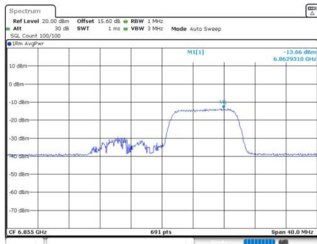
11AX20MIMO_Ant2_6855_106Tone_RU53
