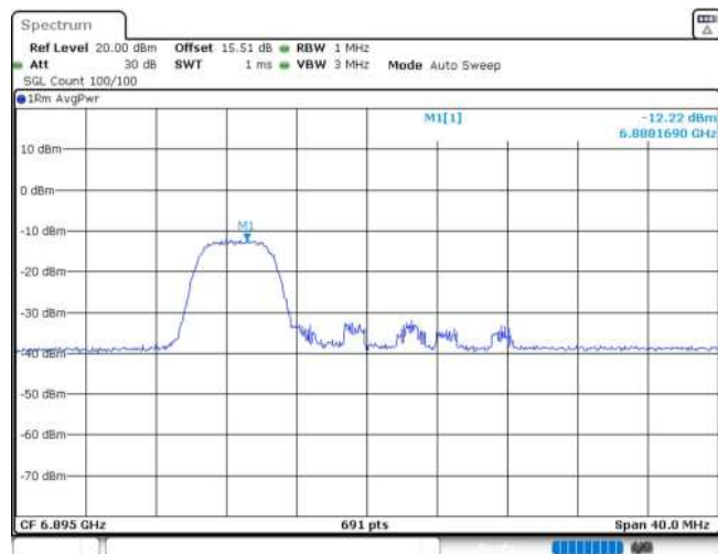
11AX20MIMO_Ant1_6895_52Tone_RU37
