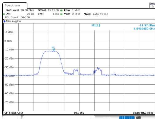
11AX20MIMO_Ant1_6855_52Tone_RU37
