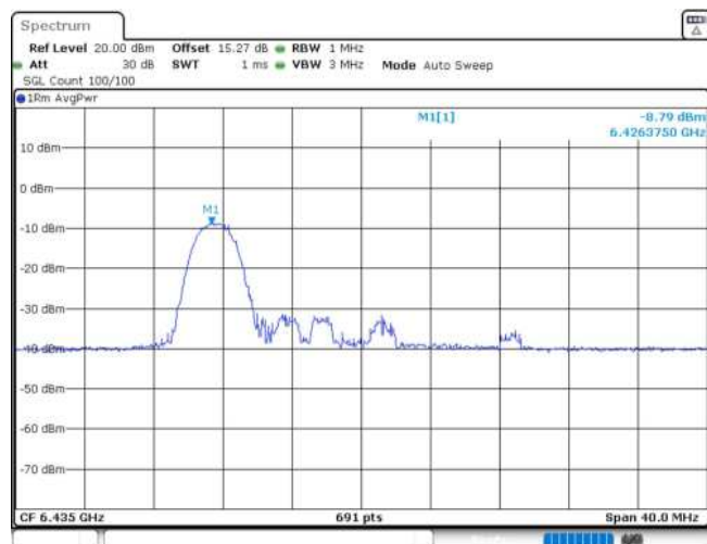
11AX20MIMO_Ant1_6435_26Tone_RU0
