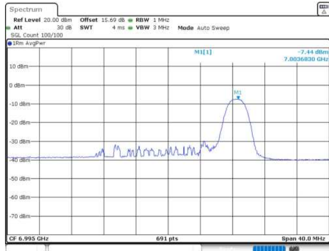
11AX20MIMO_Ant2_6995_26Tone_RU8
