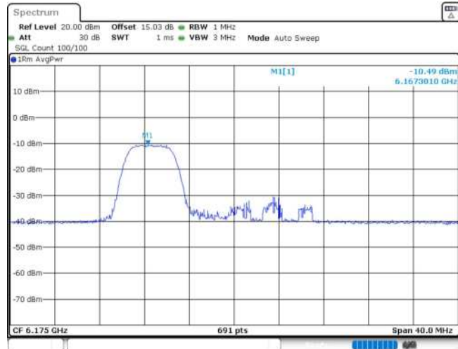
11AX20MIMO_Ant2_6175_52Tone_RU37
