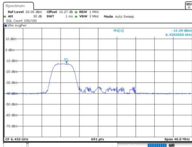
11AX20MIMO_Ant1_6435_52Tone_RU37
