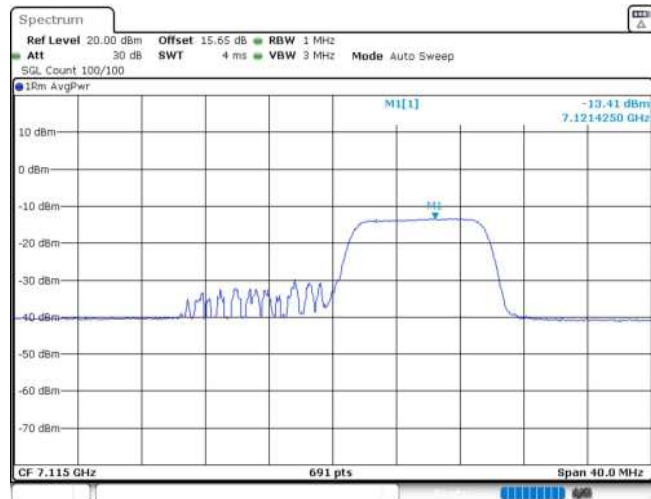
11AX20MIMO_Ant2_7115_106Tone_RU54
