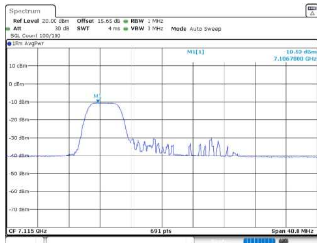
11AX20MIMO_Ant2_7115_26Tone_RU8
