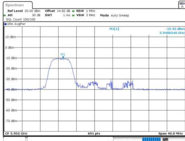
11AX20MIMO_Ant2_5955_52Tone_RU37
