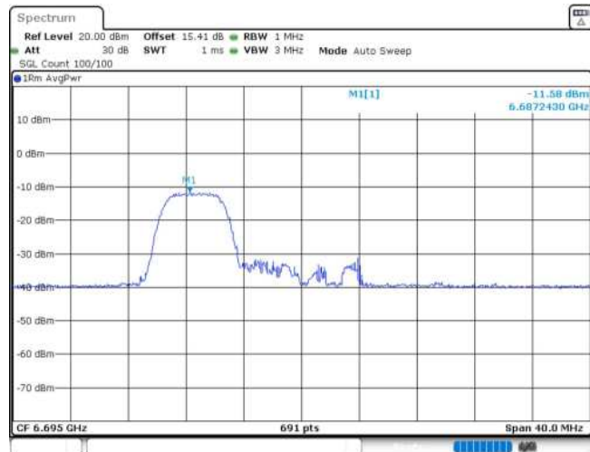
11AX20MIMO_Ant1_6695_52Tone_RU37
