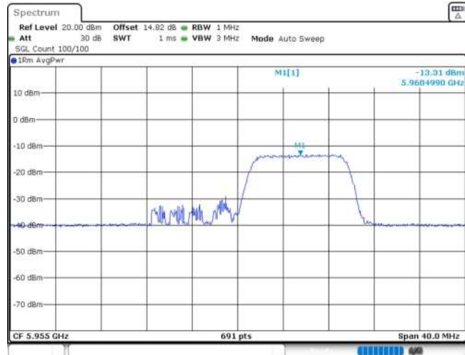
11AX20MIMO_Ant2_5955_106Tone_RU54
