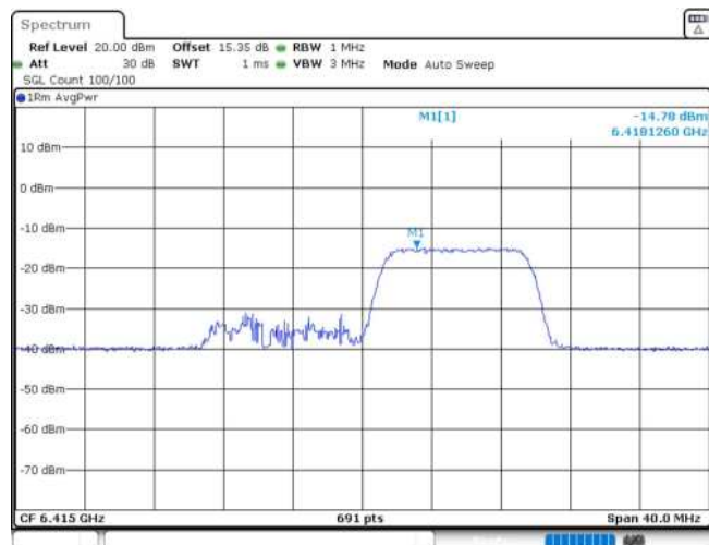
11AX20MIMO_Ant2_6415_106Tone_RU53
