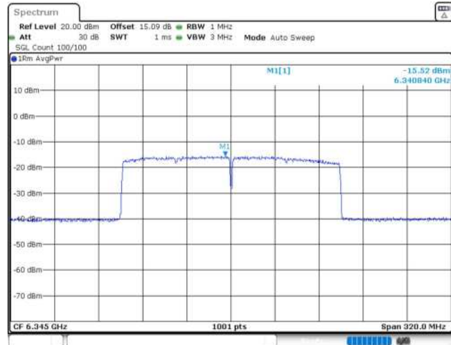
11AX160MIMO_Ant1_6345
