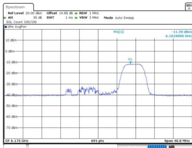
11AX20MIMO_Ant1_6175_52Tone_RU40
