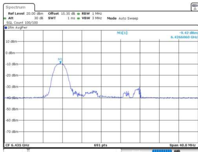
11AX20MIMO_Ant1_6435_106Tone_RU54
