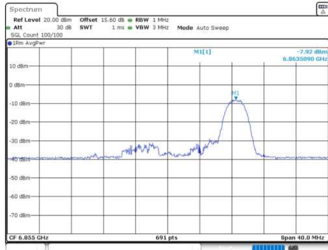
11AX20MIMO_Ant2_6855_26Tone_RU8
