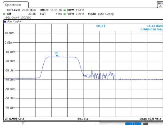
11AX20MIMO_Ant1_6995_106Tone_RU53
