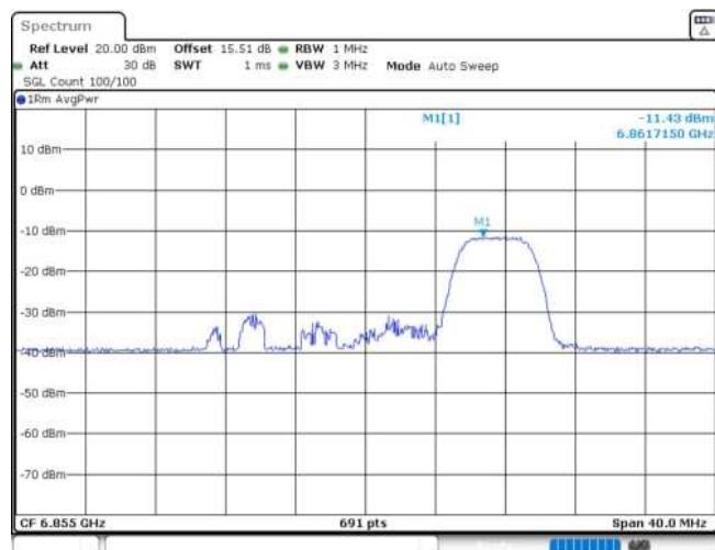
11AX20MIMO_Ant1_6855_52Tone_RU40
