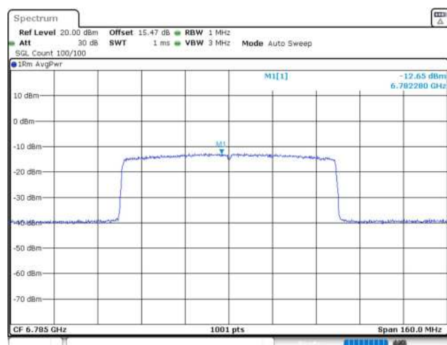
11AX80MIMO_Ant1_6785
