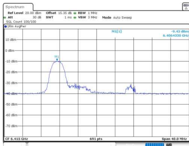
11AX20MIMO_Ant2_6415_26Tone_RU0
