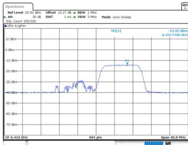
11AX20MIMO_Ant1_6415_106Tone_RU54
