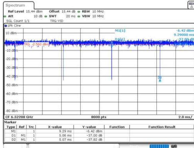
11AX20MIMO_Ant1_6515_52Tone_RU40
