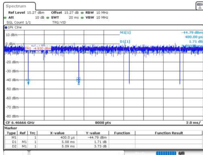
11AX20MIMO_Ant1_6475_26Tone_RU0
