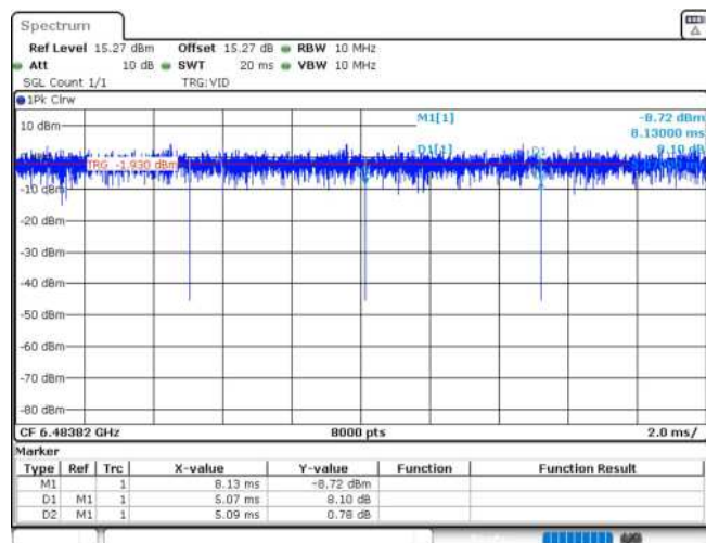
11AX20MIMO_Ant1_6475_26Tone_RU8
