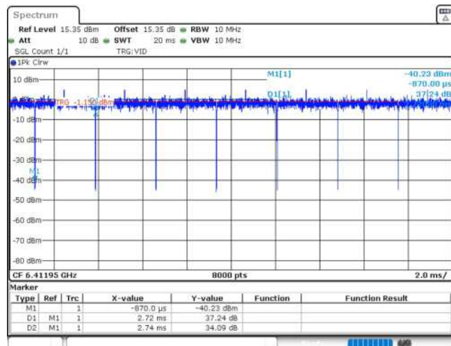
11AX20MIMO_Ant2_6415_52Tone_RU40
