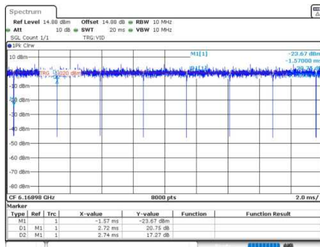
11AX20MIMO_Ant1_6175_52Tone_RU40
