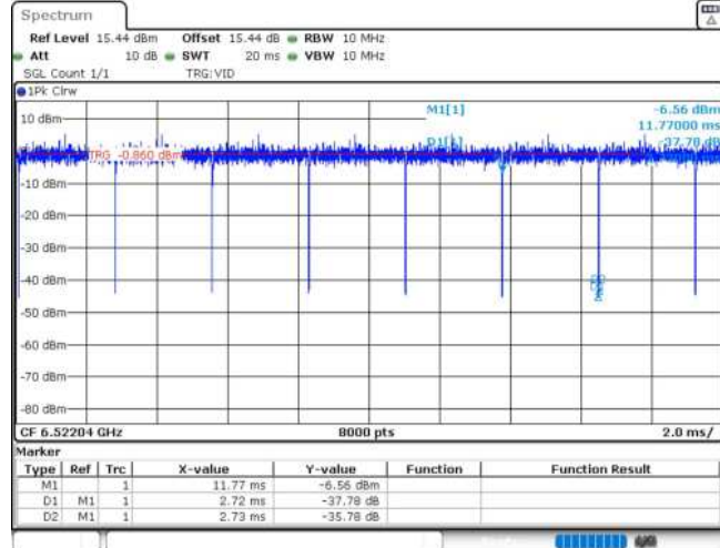
11AX20MIMO_Ant1_6515_106Tone_RU54
