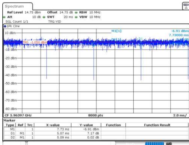
11AX20MIMO_Ant1_5955_26Tone_RU0
