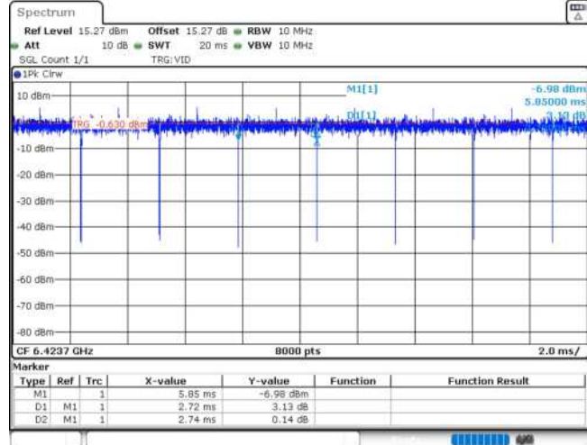
11AX20MIMO_Ant1_6415_106Tone_RU54
