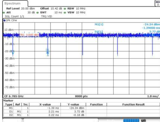
11AX80MIMO_Ant1_6785
