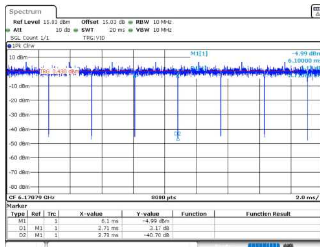
11AX20MIMO_Ant2_6175_52Tone_RU40
