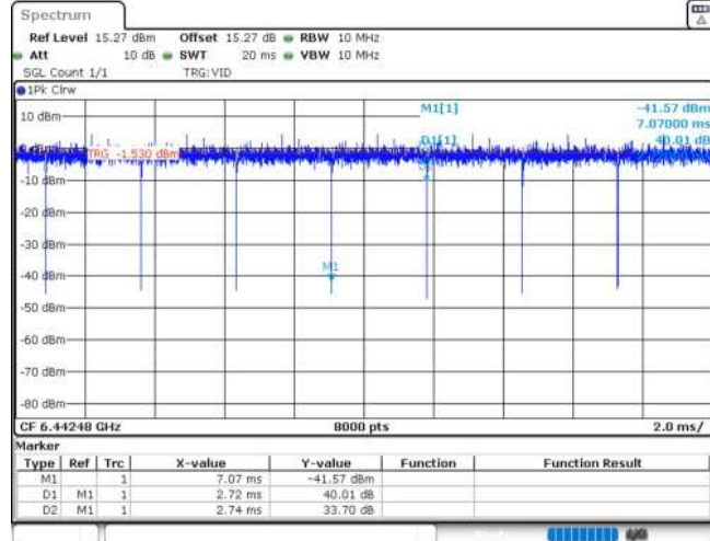
11AX20MIMO_Ant1_6435_106Tone_RU54
