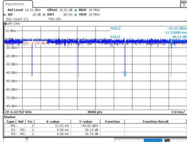
11AX20MIMO_Ant2_6535_52Tone_RU37
