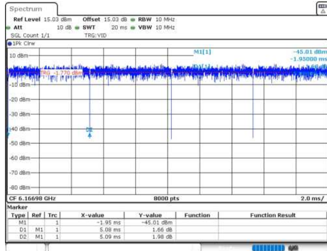
11AX20MIMO_Ant2_6175_26Tone_RU0
