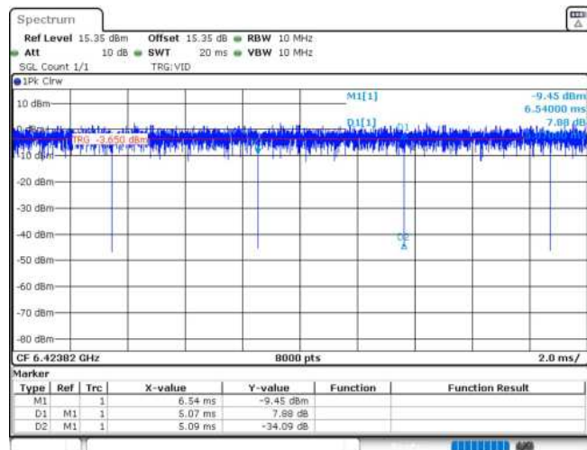
11AX20MIMO_Ant2_6415_26Tone_RU8
