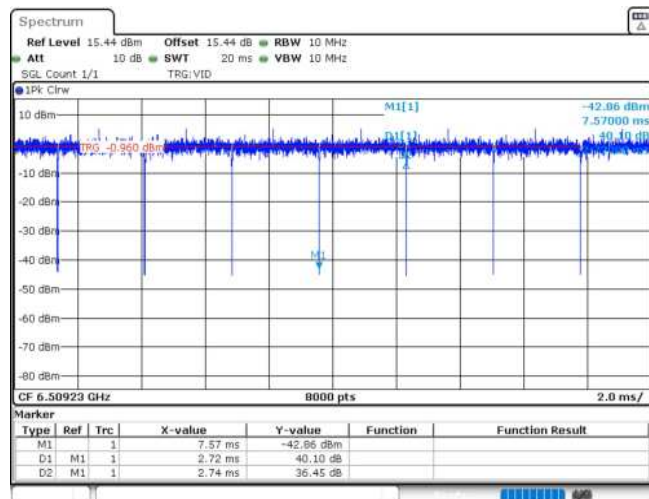
11AX20MIMO_Ant1_6515_52Tone_RU40
