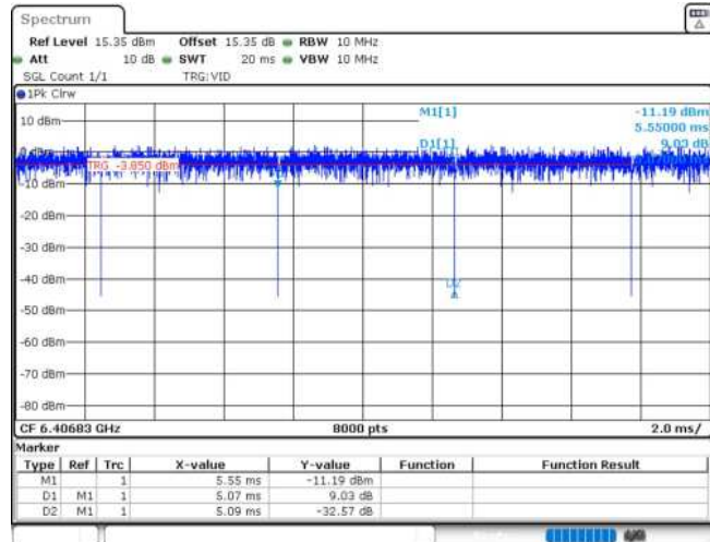
11AX20MIMO_Ant2_6415_26Tone_RU0
