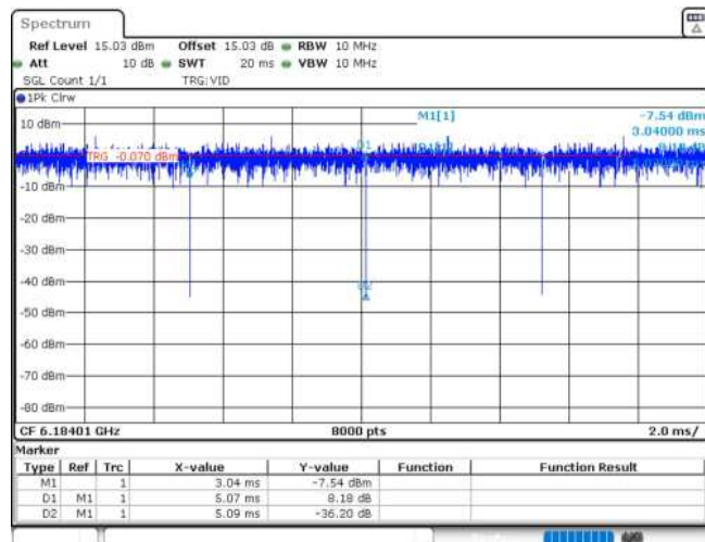
11AX20MIMO_Ant2_6175_26Tone_RU8
