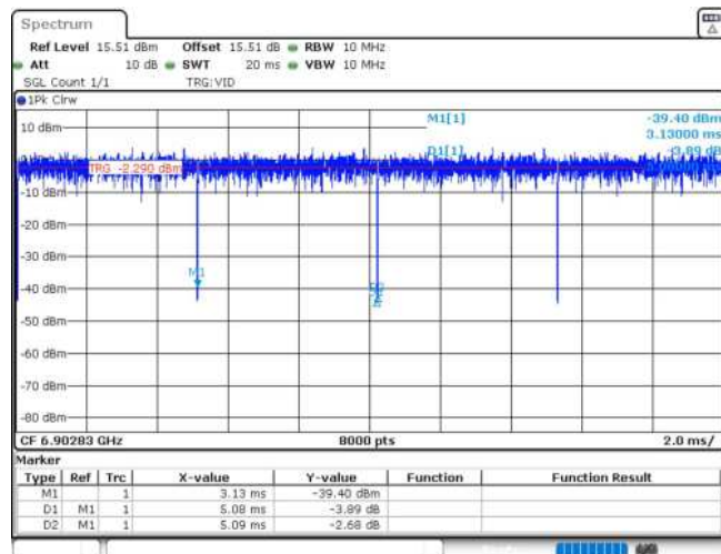
11AX20MIMO_Ant1_6895_26Tone_RU8
