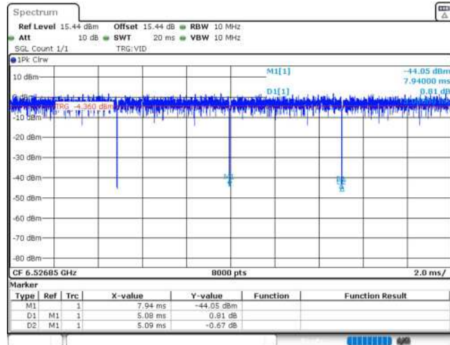
11AX20MIMO_Ant1_6535_26Tone_RU0
