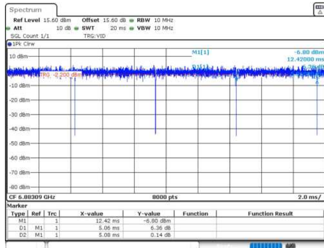
11AX20MIMO_Ant2_6875_52Tone_RU40
