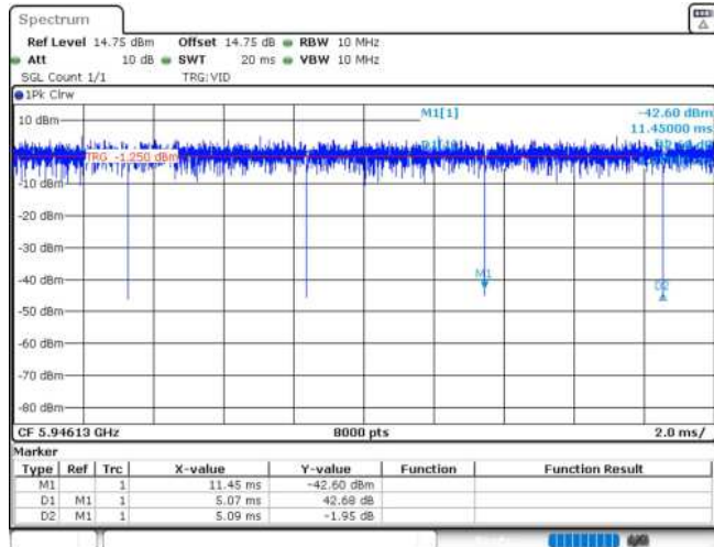
11AX20MIMO_Ant1_5955_26Tone_RU0
