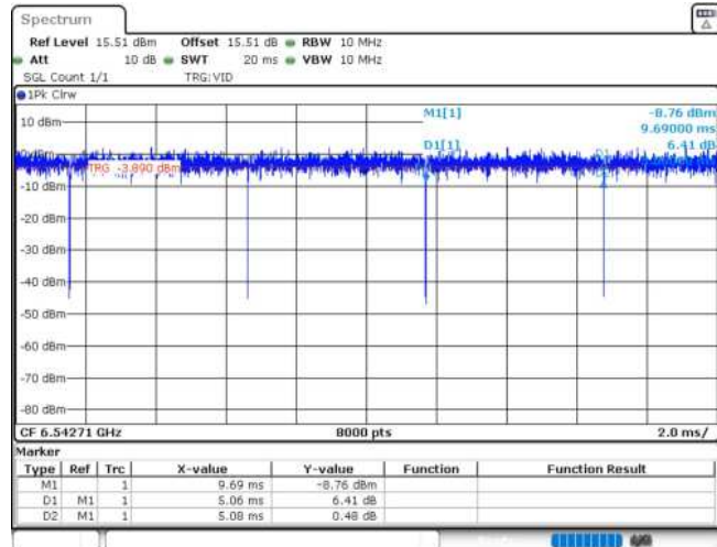
11AX20MIMO_Ant2_6535_52Tone_RU40
