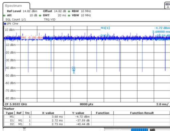
11AX20MIMO_Ant2_5955_106Tone_RU53
