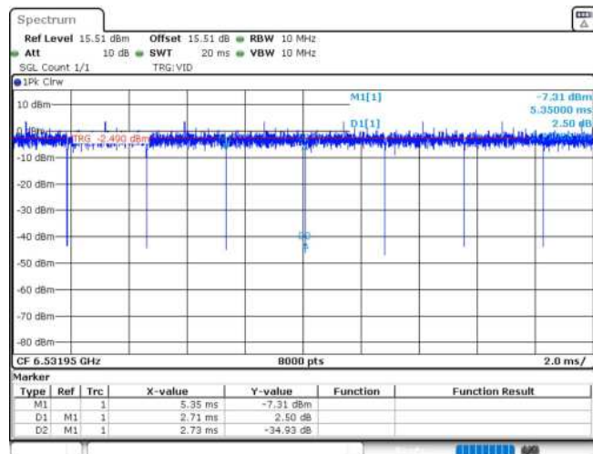
11AX20MIMO_Ant2_6535_106Tone_RU53
