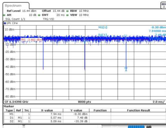
11AX20MIMO_Ant1_6535_26Tone_RU8
