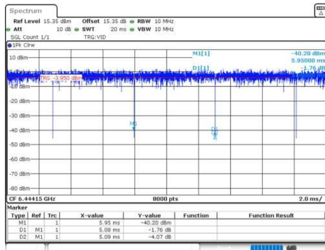
11AX20MIMO_Ant2_6435_26Tone_RU8
