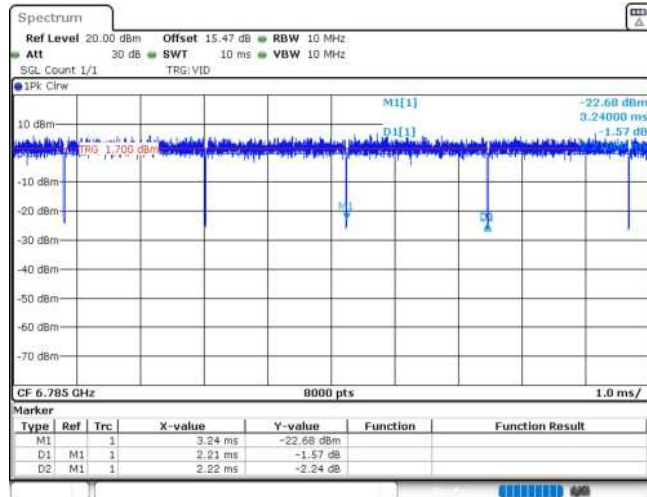
11AX80MIMO_Ant2_6785
