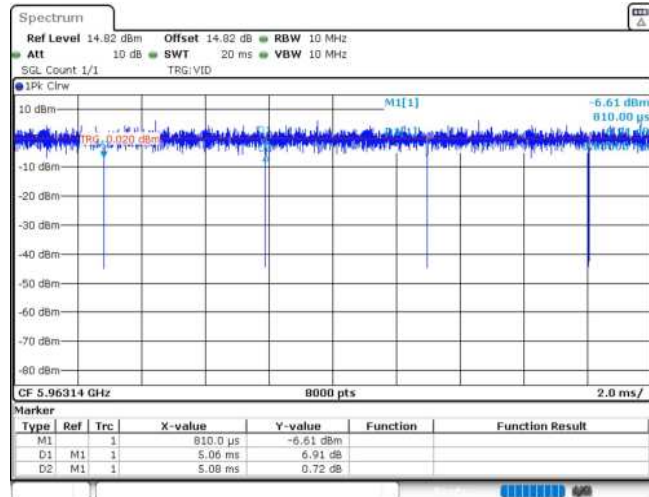
11AX20MIMO_Ant2_5955_52Tone_RU40
