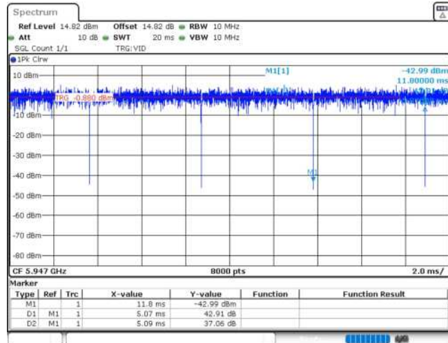
11AX20MIMO_Ant2_5955_26Tone_RU0
