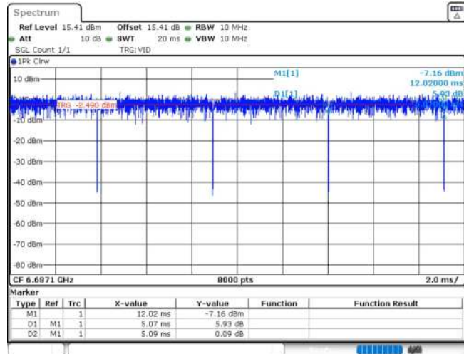
11AX20MIMO_Ant1_6695_26Tone_RU0
