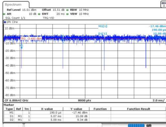
11AX20MIMO_Ant1_6895_26Tone_RU0
