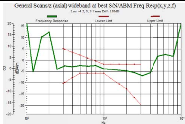
Fig 7.1 CDMA2000 BC1 Ch600
