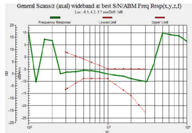
Fig. 7.4 WCDMA Band II Ch9400
