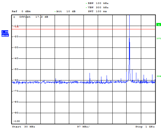
GSM 850 CH-Low 30MHz ~ 1GHz
