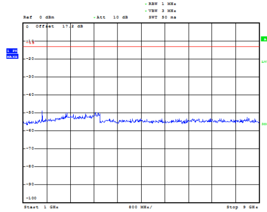
GSM 850 CH-Low 1GHz ~ 9GHz
