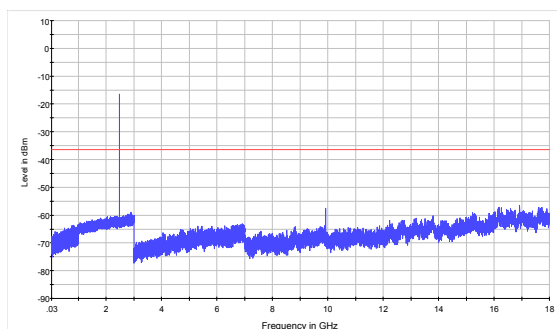
EDR-CH78 30MHz to 18GHz
