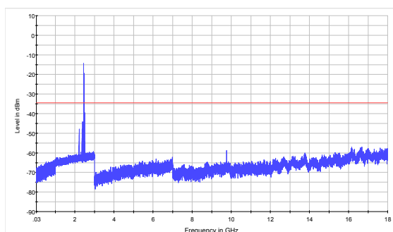
GFSK-CH78 30MHz to 18GHz
