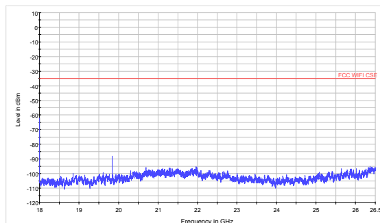
EDR-CH018GHz to 26.5GHz
