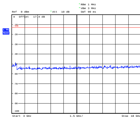
WCDMA Band IV CH-Low 3GHz~18GHz
