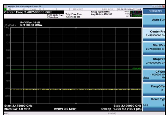
FDD07_20MHz_2560_QPSK_OneRB_low _ExtraBands_Range_2475~2490
