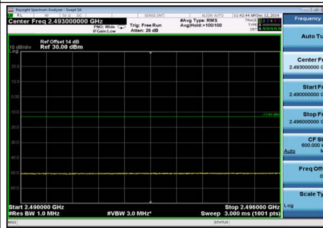
FDD07_20MHz_2560_QPSK_fullIRB_ExtraBan ds_Range_2490~2496
