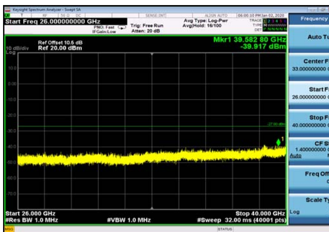
U-NII-3 ,Plot 5,26000MHz~40000MHz-802.11ac(40MHz),5755MHz,Ant1
