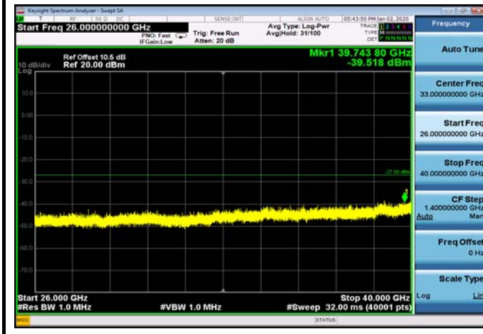
U-NII-1 ,Plot 4,26000MHz~40000MHz-802. 11ac(80MHz),5210MHz,Ant1
