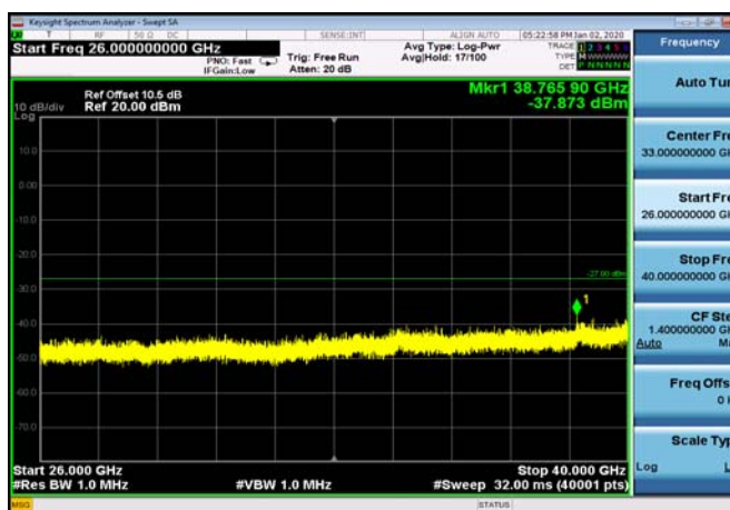
U-NII-1 ,Plot 4,26000MHz~40000MHz-802. 11ac(20MHz),5240MHz,Ant1
