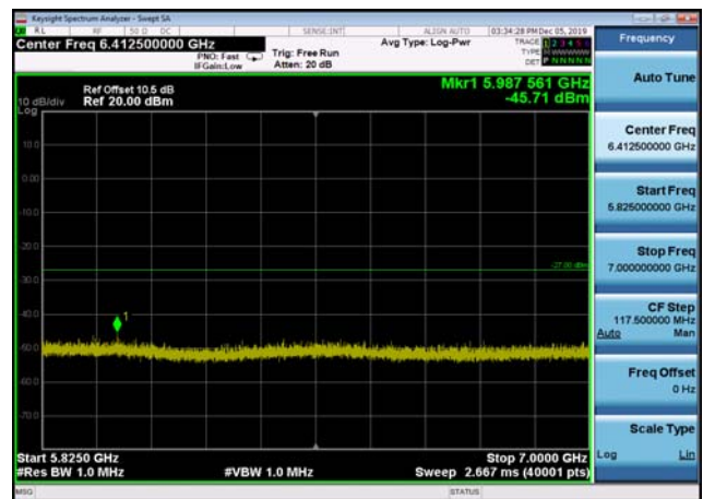
U-NII-1 ,Plot 3,5825MHz~7000MHz-802.1 1ac(20MHz),5180MHz,Ant1
