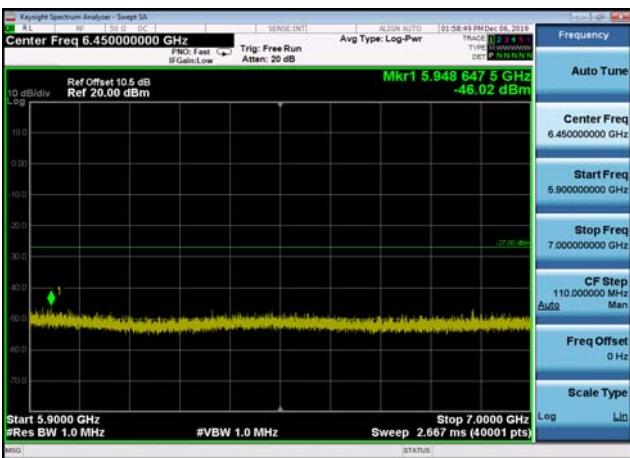
U-NII-3 ,Plot 3,5900MHz~7000MHz-802.1 n(40MHz),5755MHz,Ant1
