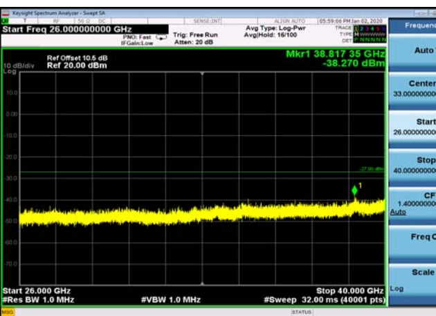
U-NII-3 ,Plot 5,26000MHz~40000MHz-802.11a (20MHz),5745MHz,Ant1
