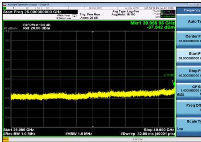
U-NII-3 ,Plot 5,26000MHz~40000MHz-802.11ac(20MHz),5785MHz,Ant1
