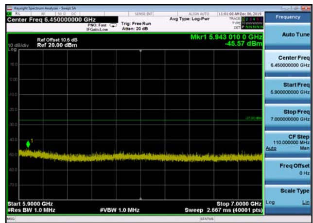
U-NII-3 ,Plot 3,5900MHz~7000MHz-802.1 1ac(40MHz),5795MHz,Ant1
