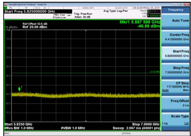
U-NII-1 ,Plot 3,5825MHz~7000MHz-802.1 1ac(40MHz),5230MHz,Ant1
