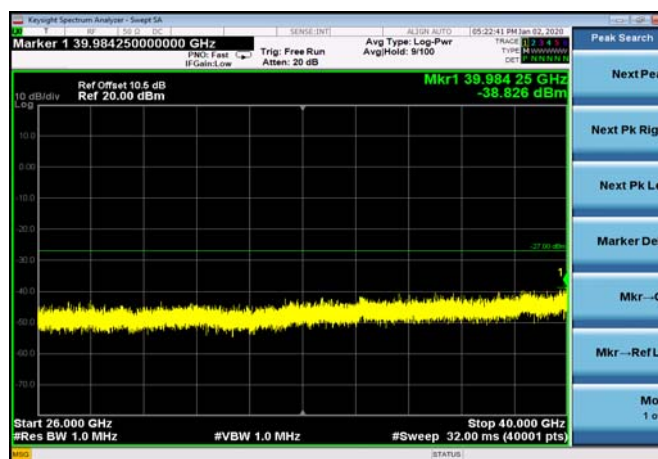
U-NII-1 ,Plot 4,26000MHz~40000MHz-802. 11ac(20MHz),5220MHz,Ant1
