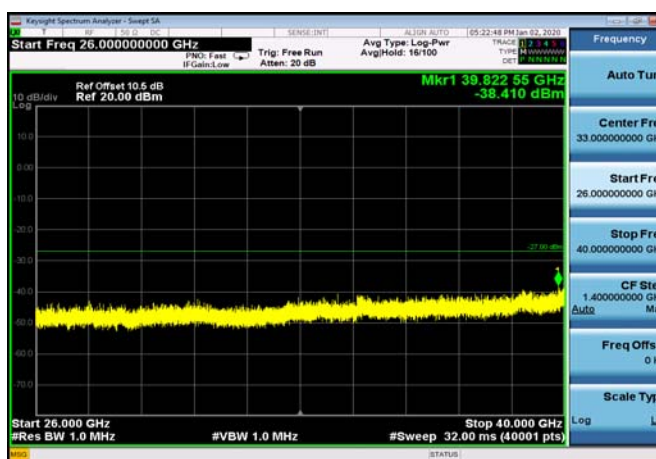
U-NII-1 ,Plot 4,26000MHz~40000MHz-802. 11ac(40MHz),5190MHz,Ant1
