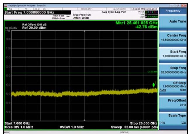
U-NII-3 ,Plot 4,7000MHz~26000MHz-802. 11n(20MHz),5745MHz,Ant1
