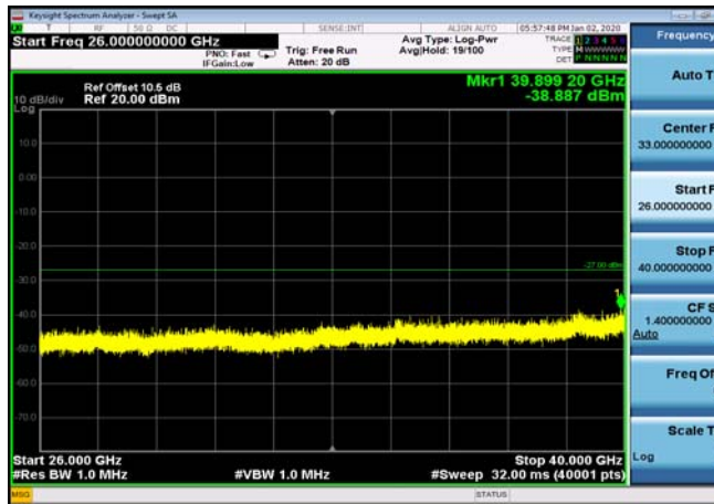
U-NII-3 ,Plot 2,26000MHz~40000MHz-802.11n (20MHz),5785MHz,Ant1
