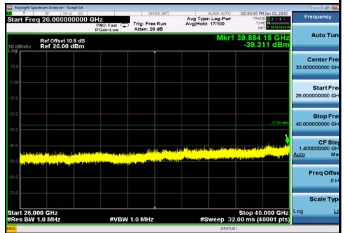
U-NII-3 ,Plot 5,26000MHz~40000MHz-802.11ac(20MHz),5825MHz,Ant1
