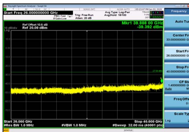
U-NII-1 ,Plot 4,26000MHz~40000MHz-802. 11ac(40MHz),5230MHz,Ant1
