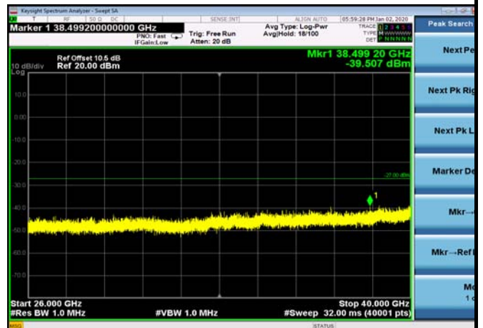
U-NII-3 ,Plot 5,26000MHz~40000MHz-802.11ac(40MHz),5795MHz,Ant1
