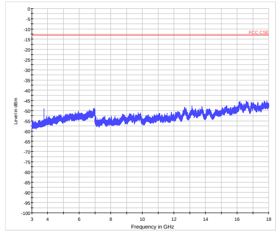
NB-IOT Band 2 CH-Middle 3GHz~18GHz
