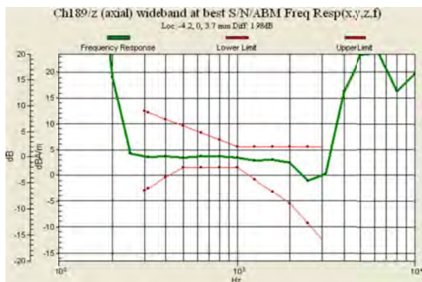
Fig 7.1 GSM850 Ch189
