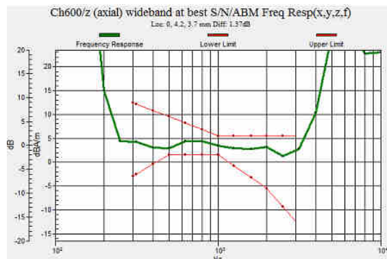
Fig 7.2 CDMA2000 BC1 Ch600
