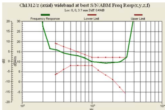
Fig. 8.11 WCDMA Band IV Ch1312
