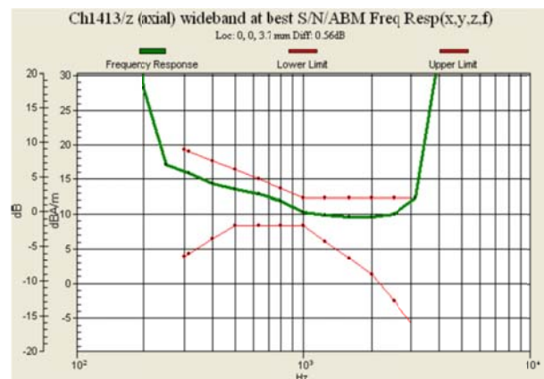
Fig. 8.12 WCDMA Band IV Ch1413
