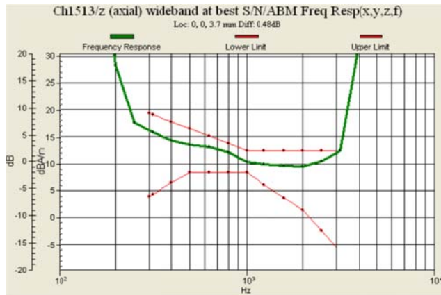
Fig. 8.13 WCDMA Band IV Ch1513
