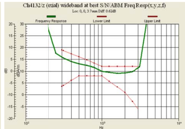
Fig. 8.8 WCDMA Band V Ch4132
