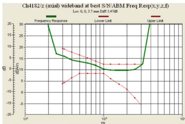
Fig. 8.9 WCDMA Band V Ch4182
