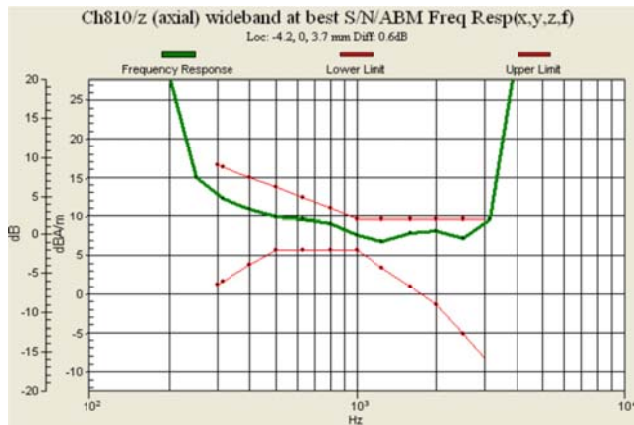
Fig 8.7 GSM1900 Ch810
