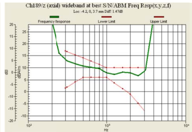
Fig 8.2 GSM850 Ch189
