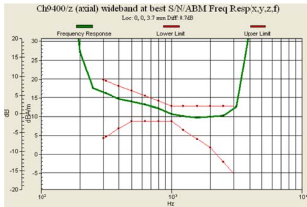
Fig. 8.15 WCDMA Band II Ch9400
