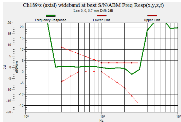
Fig 7.1 GSM850 Ch189
