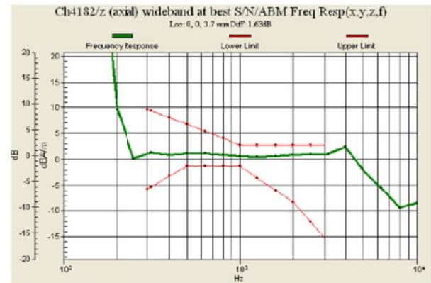
Fig. 7.8 WCDMA Band V Ch4182
