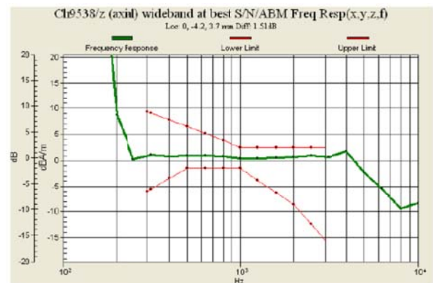
Fig. 7.12 WCDMA Band II Ch9538
