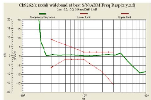
Fig. 7.10 WCDMA Band II Ch9262
