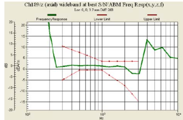
Fig 7.2 GSM850 Ch189
