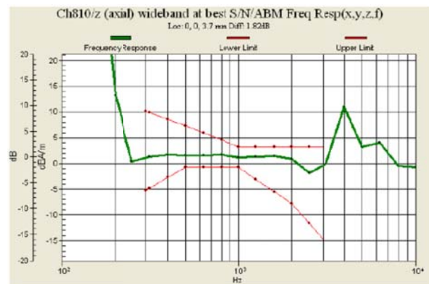
Fig 7.6 GSM1900 Ch810
